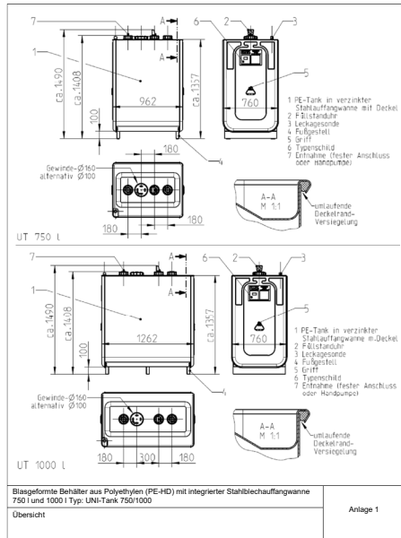
Blasgeformte Behälter aus Polyethylen (PE-HD) mit integrierter Stahltauffangwanne 750 l und 1000 l Typ: UNI-Tank 750/1000
