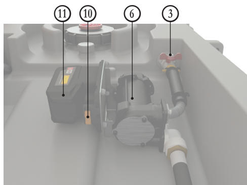
DT-Mobil Easy 460 I / 600 I avec batterie CAS
