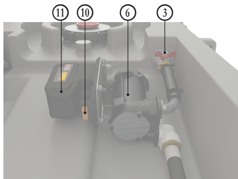
DT-Mobil Easy 460I / 600I cu acumulator CAS
