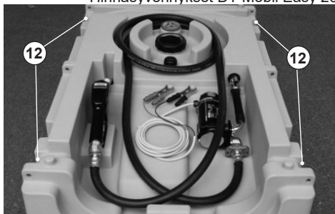
Hihnasyvennykset DT-Mobil Easy 430l
