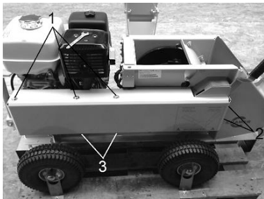
1-3 = Sechskantmuttern mit Unterlegscheibe
