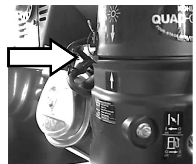
Zündkerzenstecker
