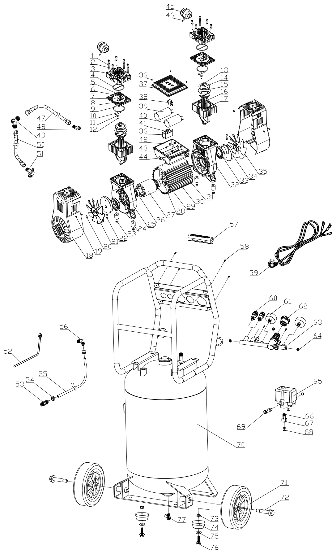
Abb. 17: Ersatzteilzeichnung COMPACT AIR 320/90 V OF E
