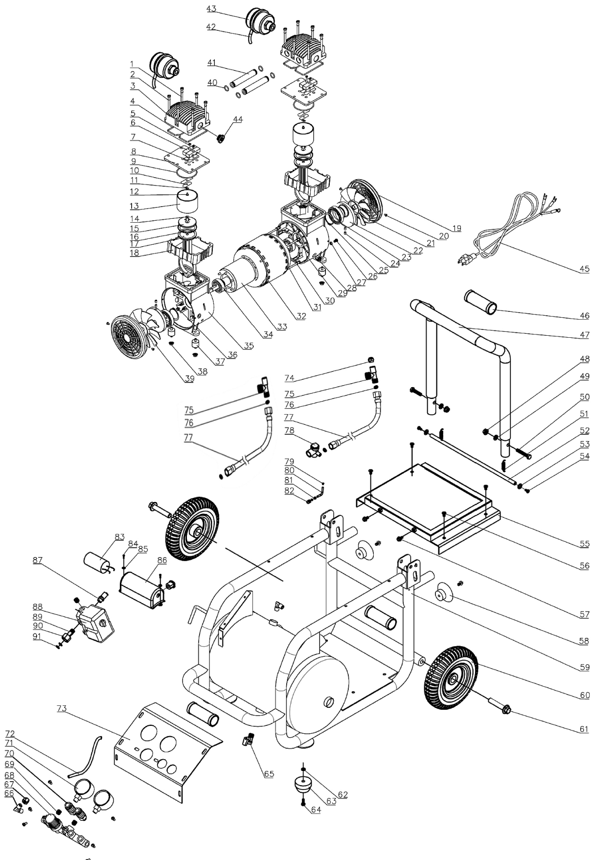
Abb. 14: Ersatzteilzeichnung COMPACT-AIR 240/20 OF E
