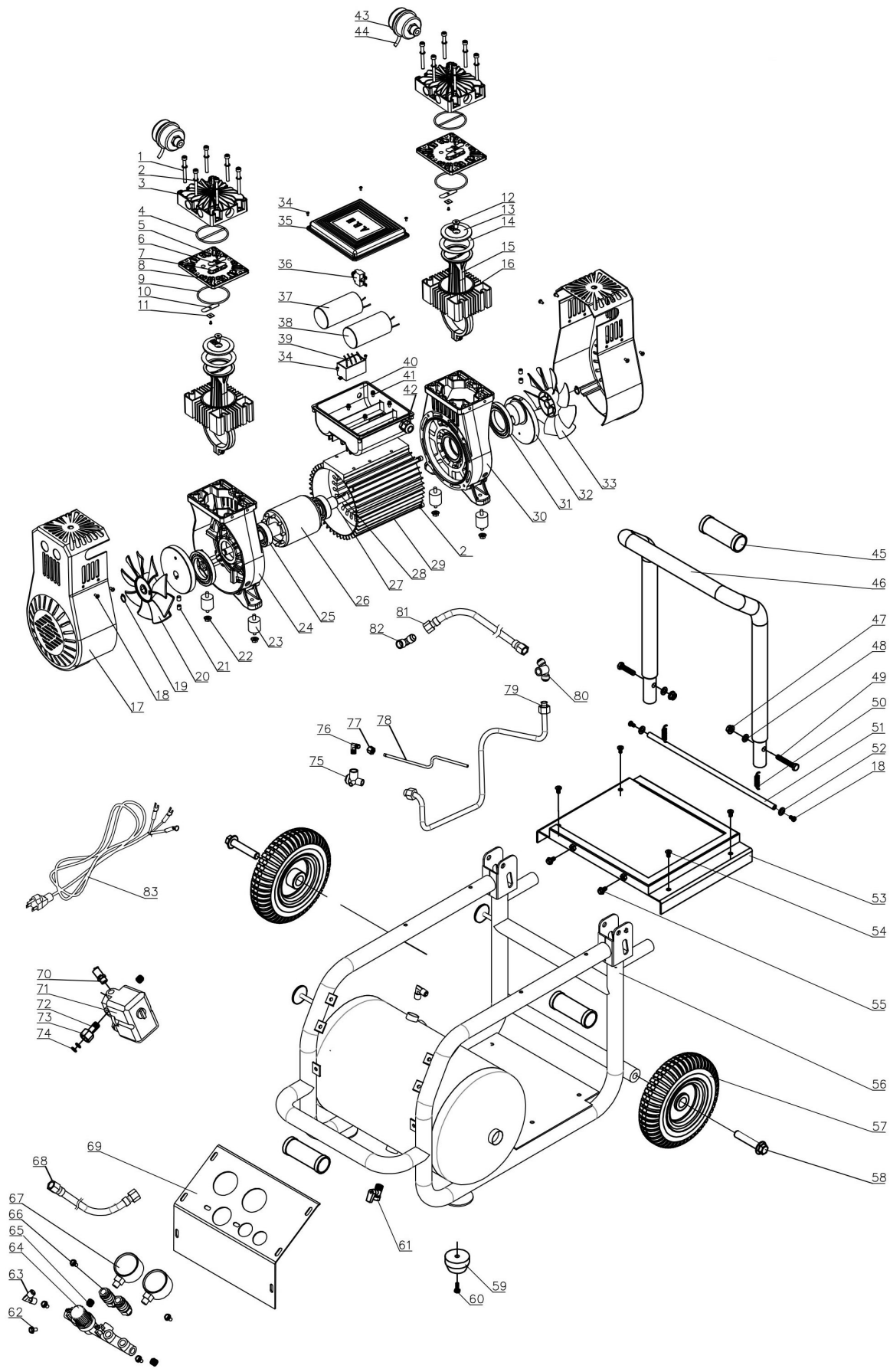
Abb. 16: Ersatzteilzeichnung COMPACT-AIR 320/24 OF E
