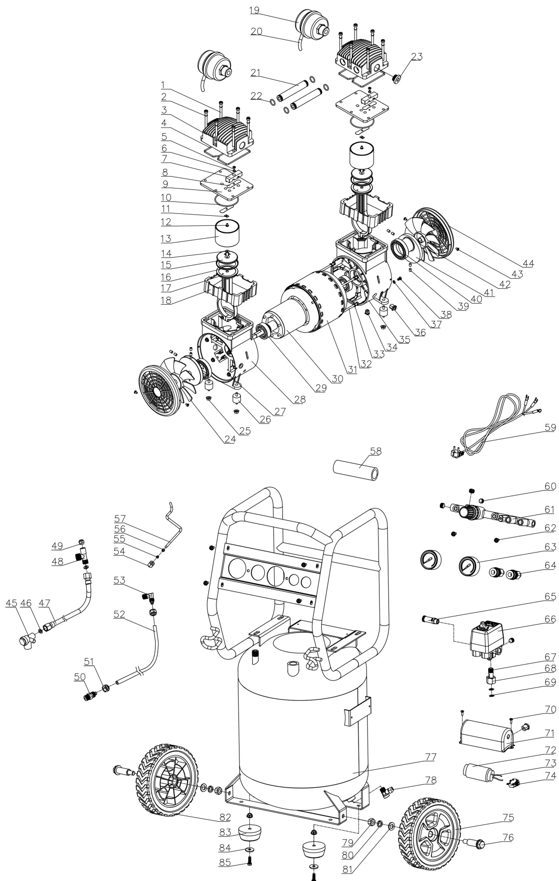
Abb. 15: Ersatzteilzeichnung COMPACT-AIR 240/40 V OF E
