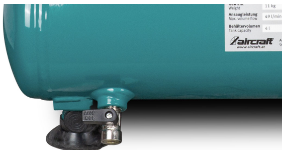
Abb. 6: Entlüftungsventil
