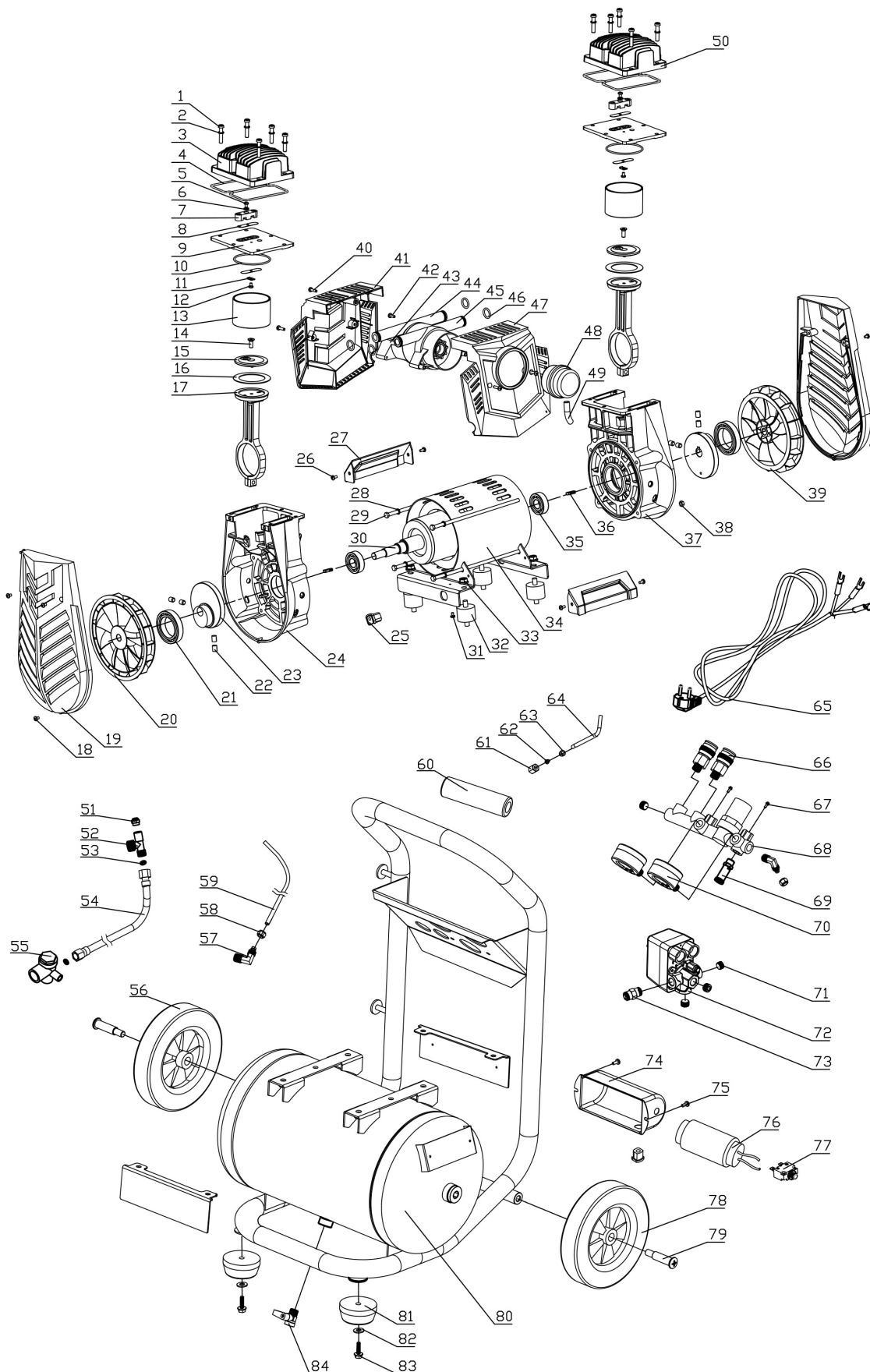
Abb. 18: Ersatzteilzeichnung COMPACT AIR 320/90 V OF E
