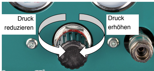
Abb. 9: Einstellen des Arbeitsdrucks
