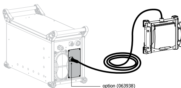
NEOPULSE/PULSEMIG 400 CW
