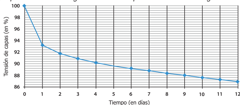
Ejemplo de la autodescarga natural de un supercondensador a lo largo del tiempo
