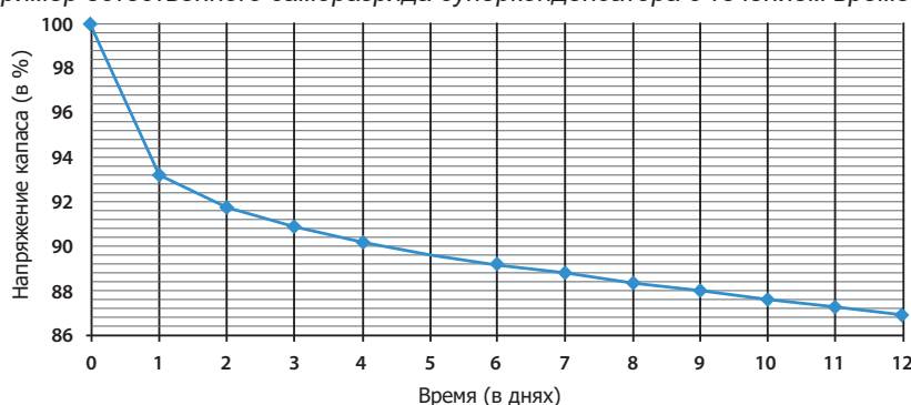
Пример естественного саморазряда суперконденсатора с течением времени
