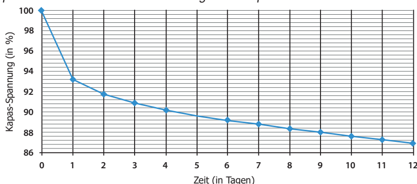
Beispiel für die natürliche Selbstentladung eines Superkondensators im Laufe der Zeit
