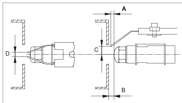
Abb. 10: Einstellen von Zündelektrode und Stauscheibe
