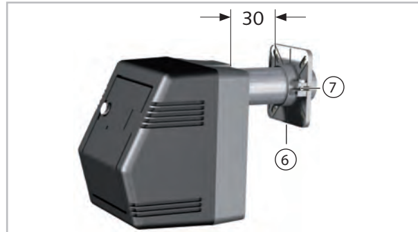
Abb. 19: Montage des Brennerflansches und des Brenners
