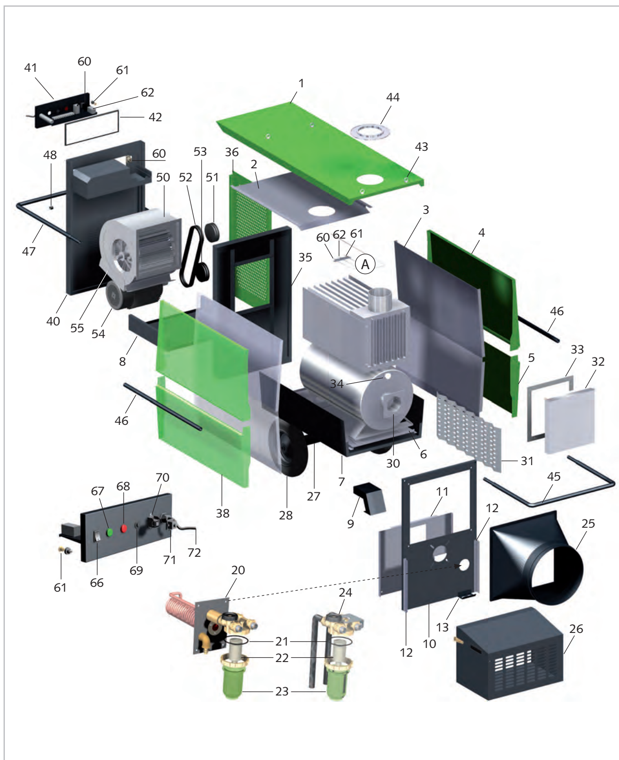
Abb. 21: Gerätedarstellung CLK 80-170-RV
