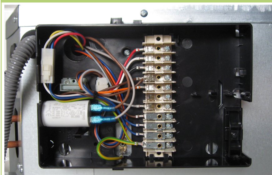
Elektrischer Anschluss
