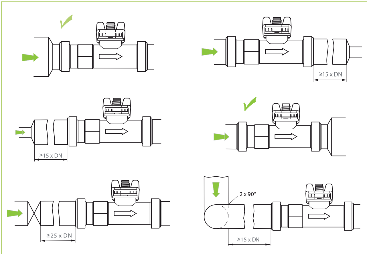
Abb. 7: Anschlussmöglichkeiten
