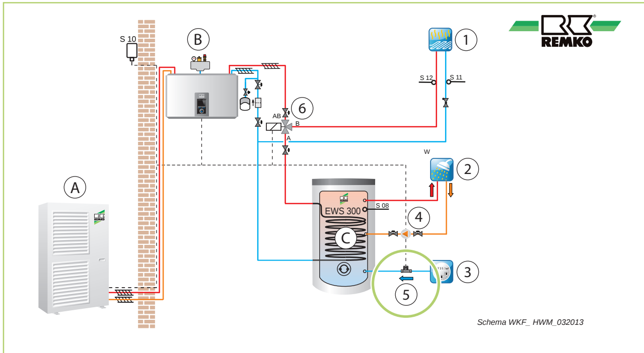
Abb. 11: Hydraulikschema 1
