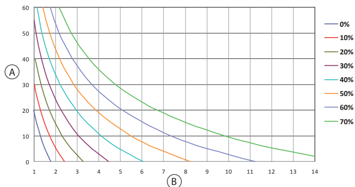
Abb. 1: Kinematische Viskosität Ethylenglykol-Wasser
