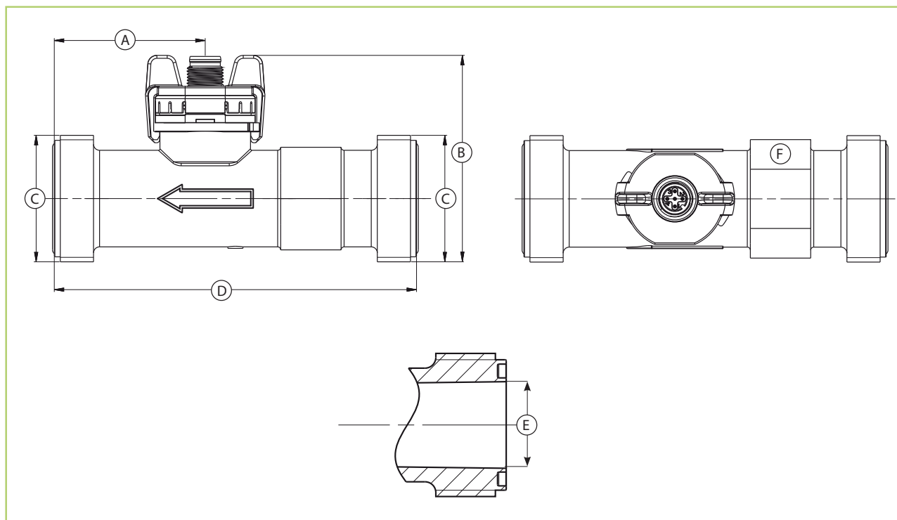
Abb. 5: Abmessungen
