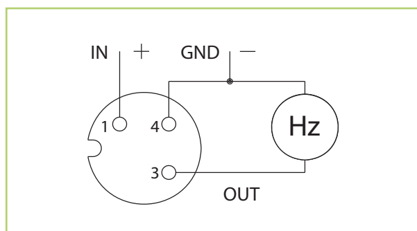
Abb. 13: Frequenzausgang
