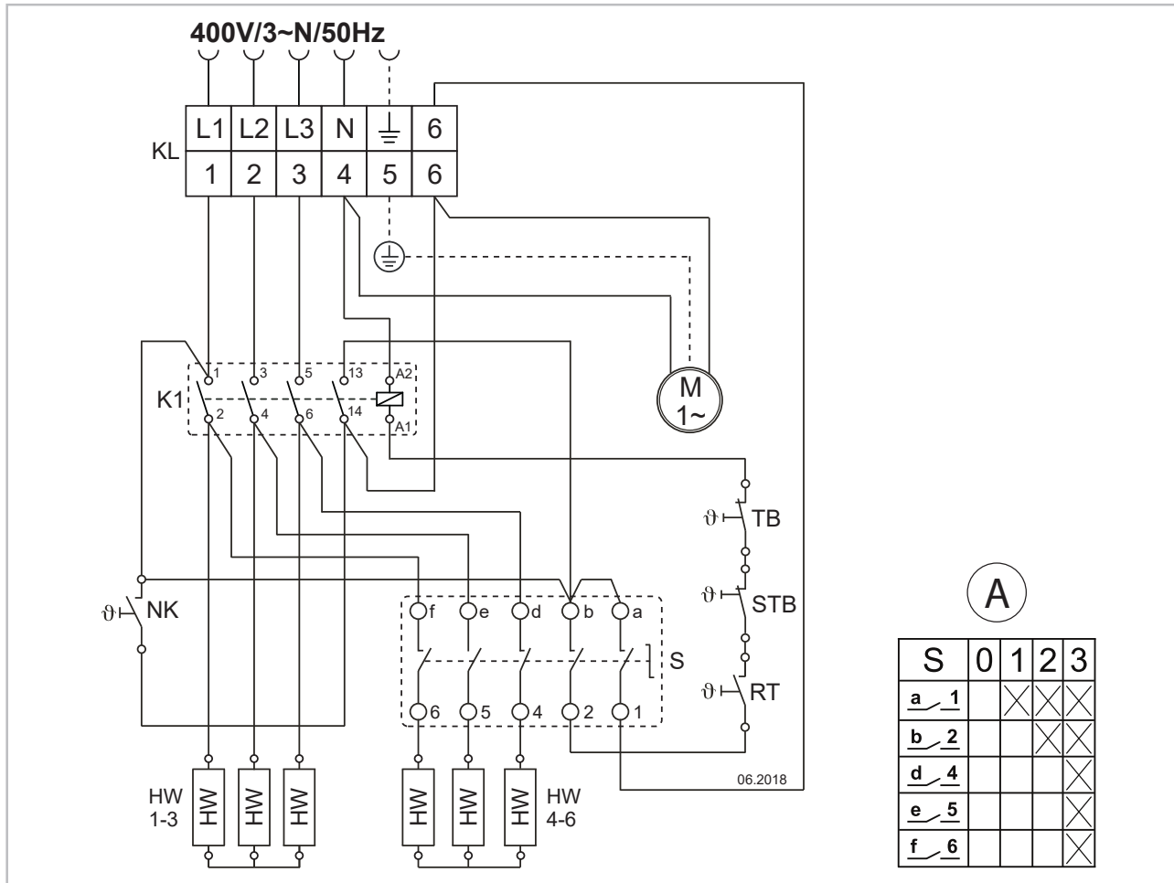
Abb. 1: Elektrisches Anschlussschema
