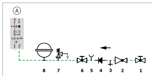
Abb. 6: Montagebeispiel
