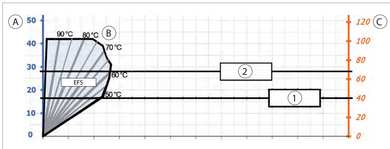
Abb. 10: Maximaler Zapfvolumenstrom
