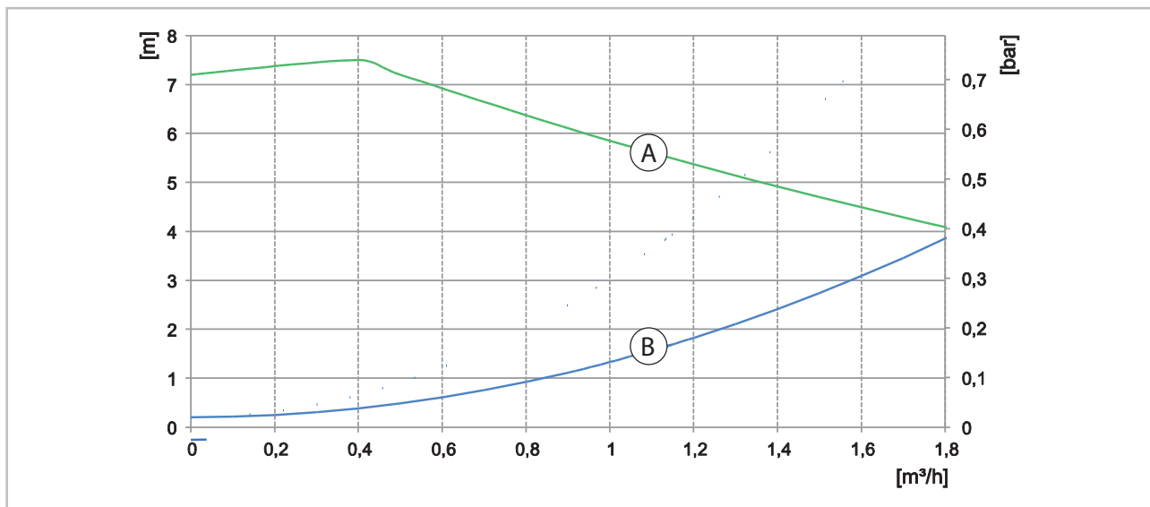
Abb. 2: Druckverlustkennlinie
