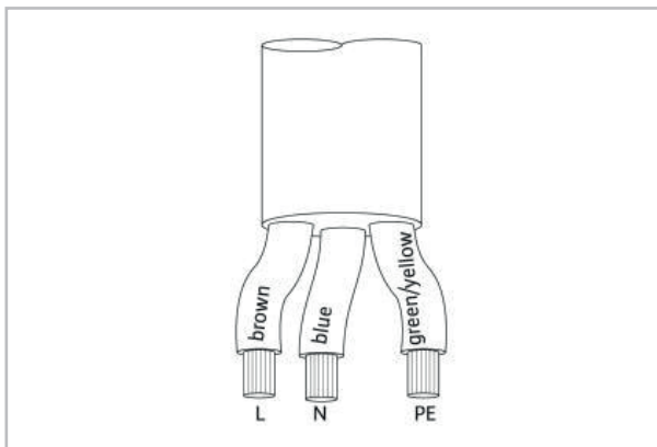
Abb. 9: Elektrischer Anschluss Pumpe
