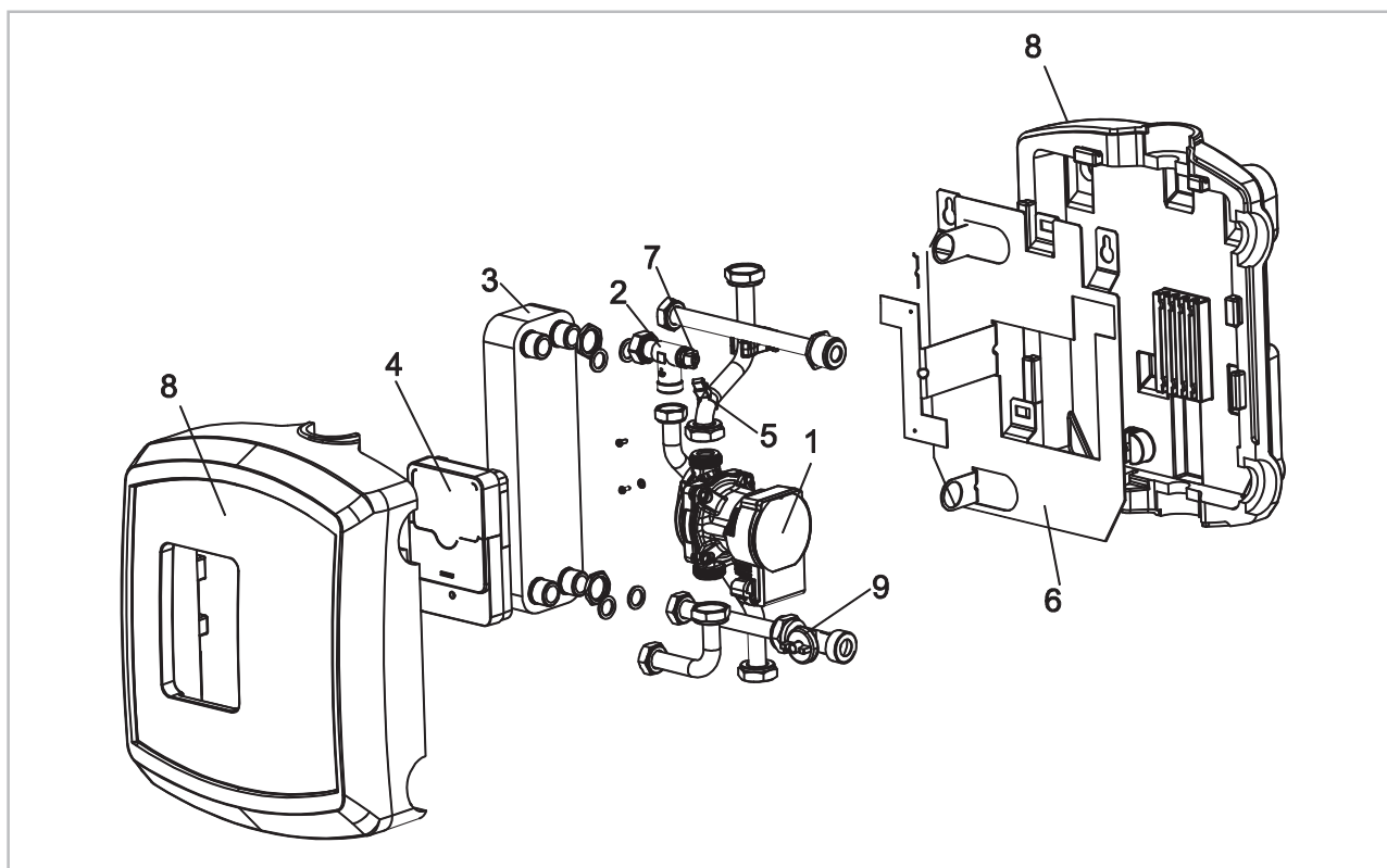
Abb. 12: Ersatzteile
