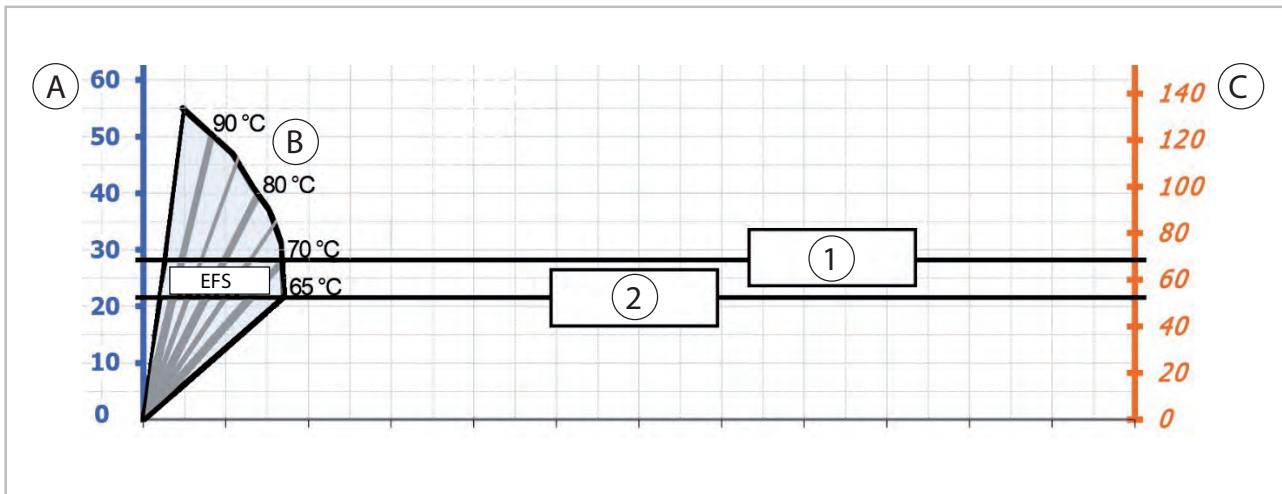
Abb. 11: Maximaler Zapfvolumenstrom
