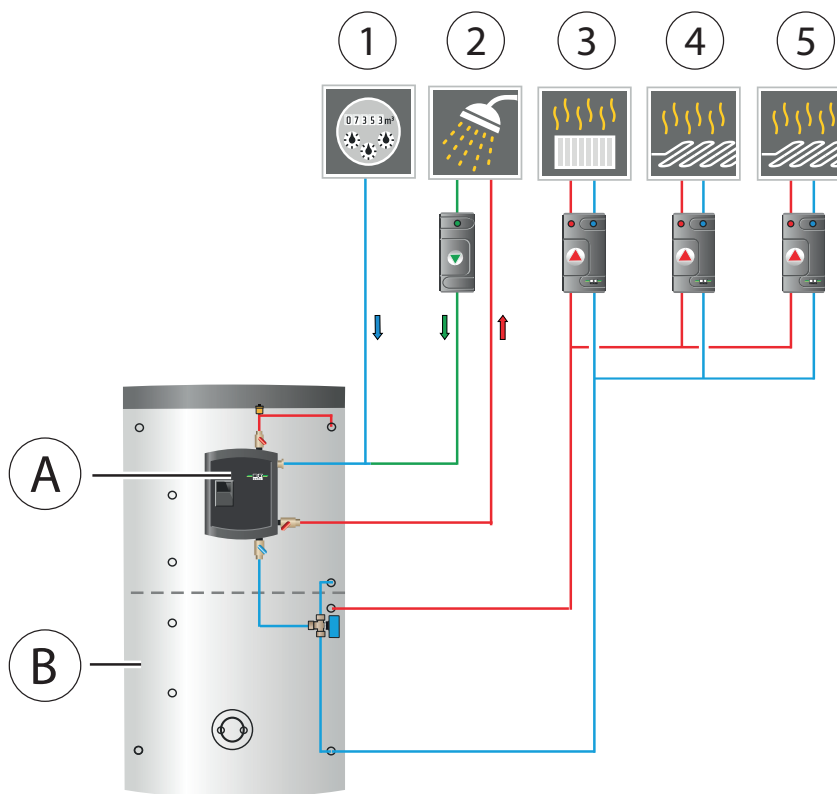
Abb. 4: Frischwasserstation mit optionalem Zirkulationsset sowie mit optionaler Rücklaufverteilung
