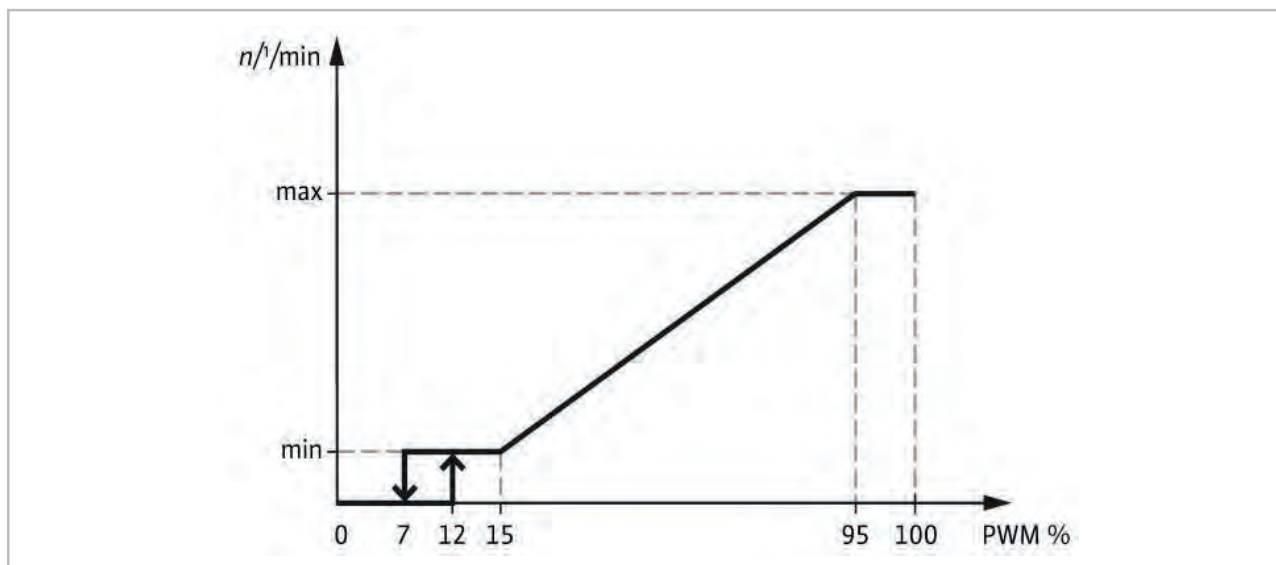
Abb. 3: PWM-Logik
