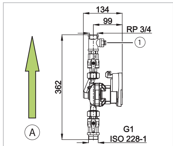
Abb. 8: Optionales Zirkulationsset
