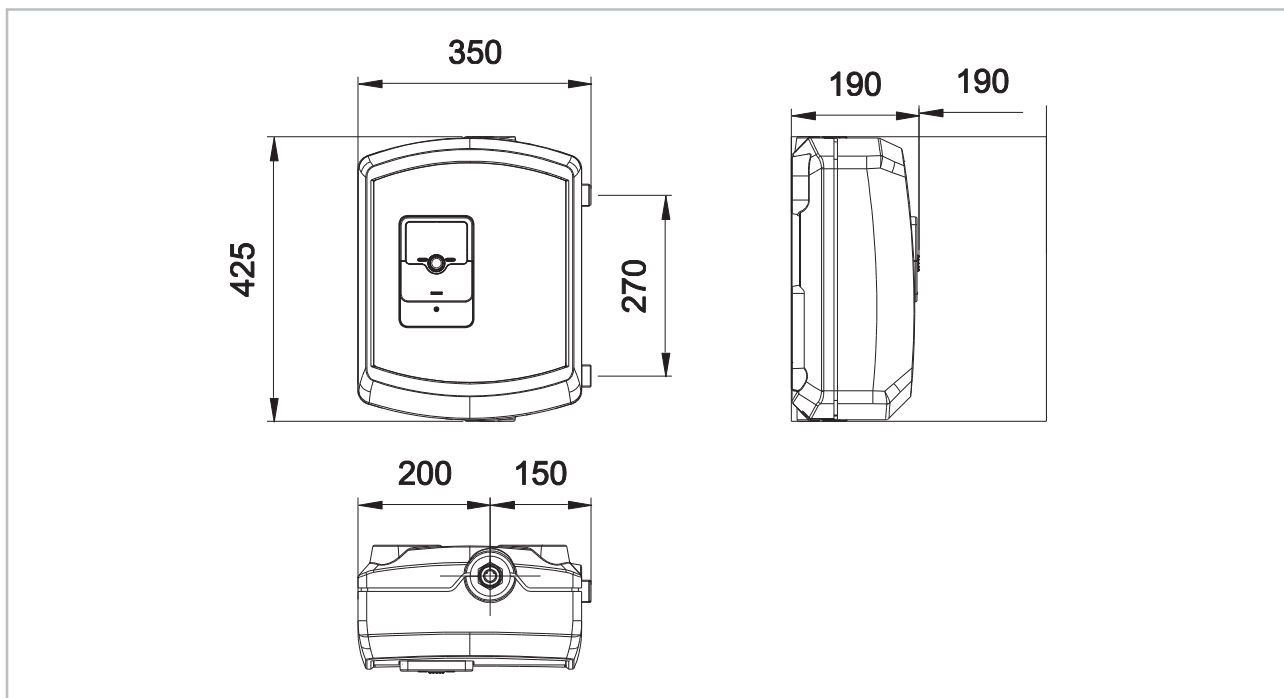
Abb. 1: Geräteabmessungen
