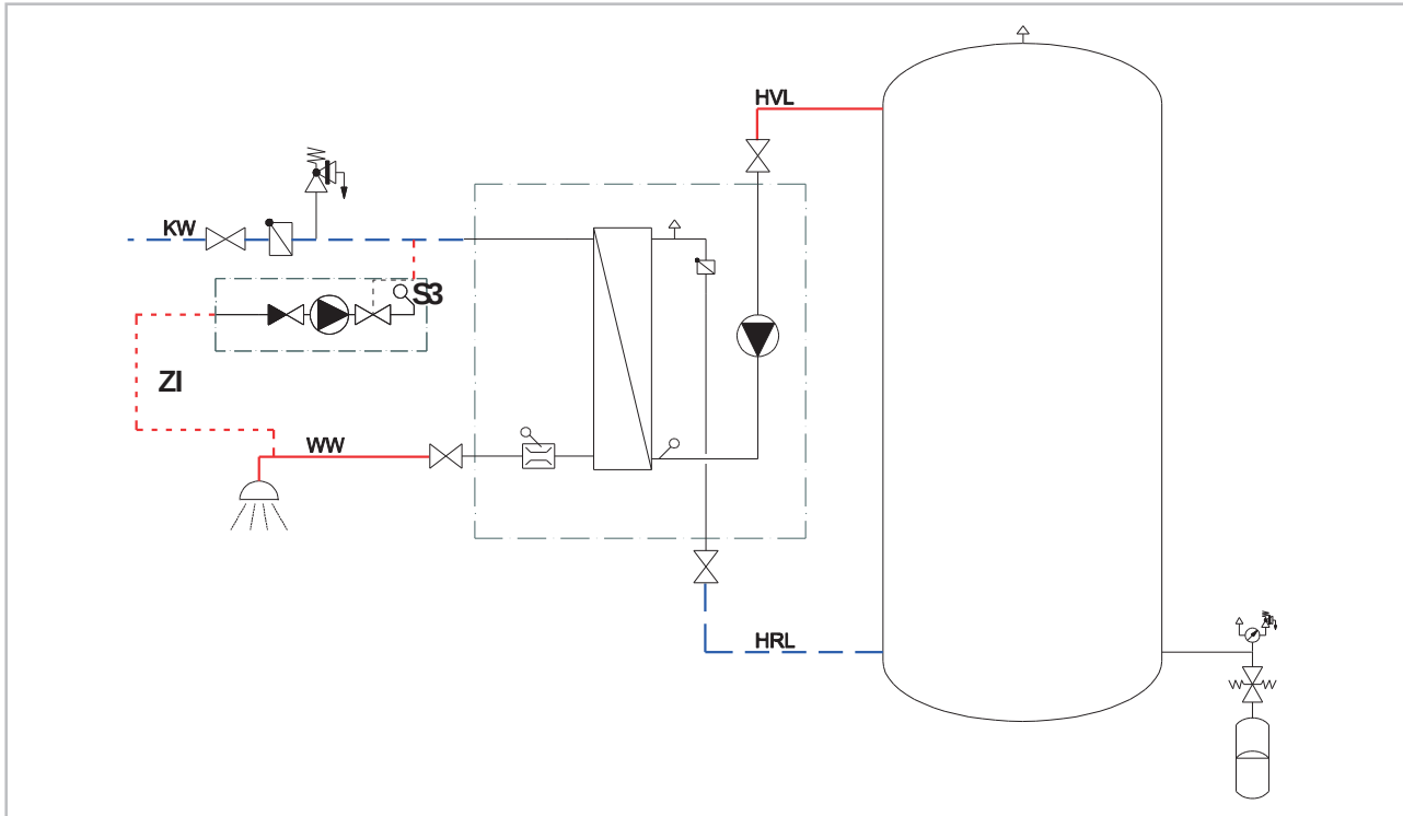
Abb. 7: Hydraulischer Anschluss
