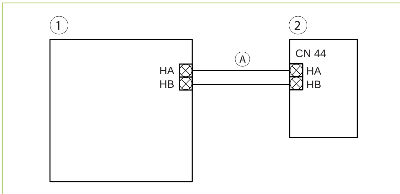
Abb. 4: Elektrisches Anschlussschema
