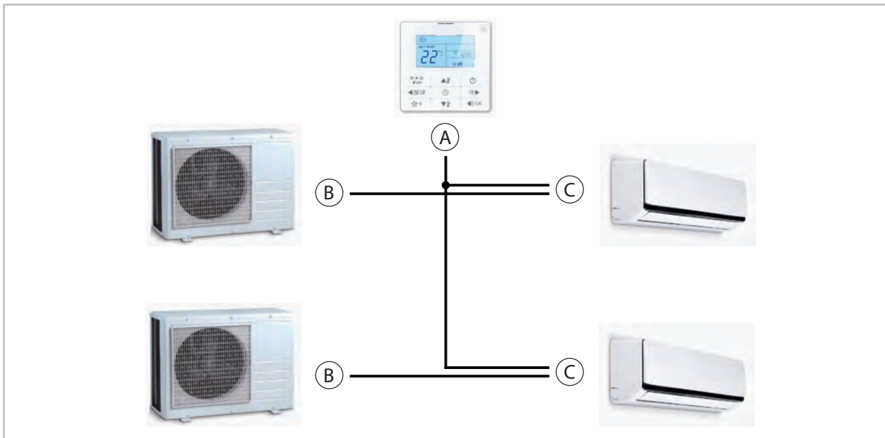
Abb. 6: Beispiel Montage zweier Singlesplitkombinationen mit einer Fernbedienung
