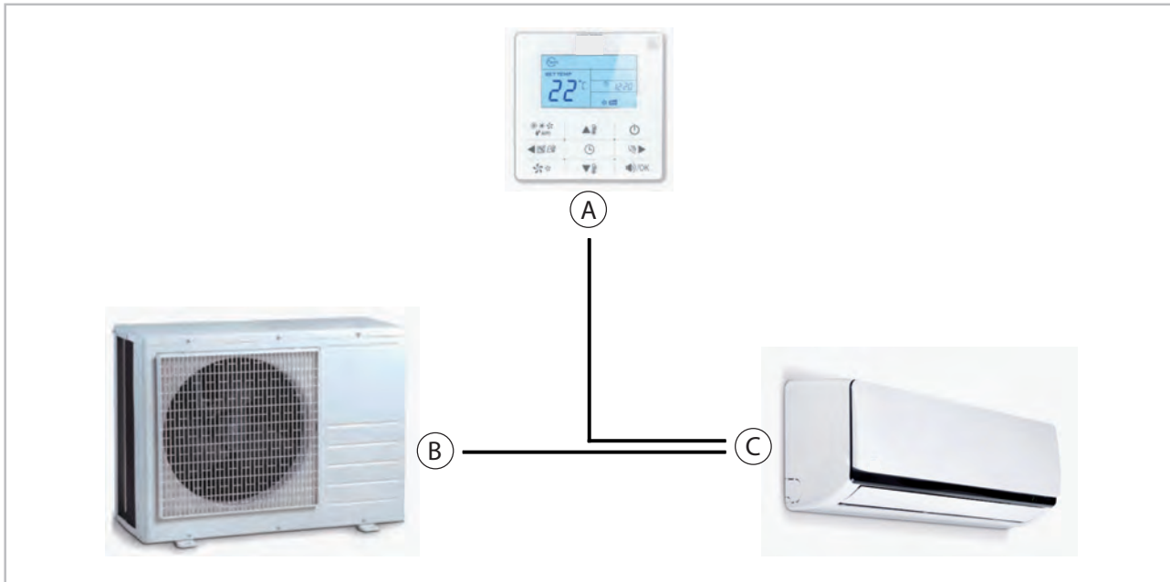
Abb. 5: Beispiel Montage Singlesplitkombination mit einer Fernbedienung
