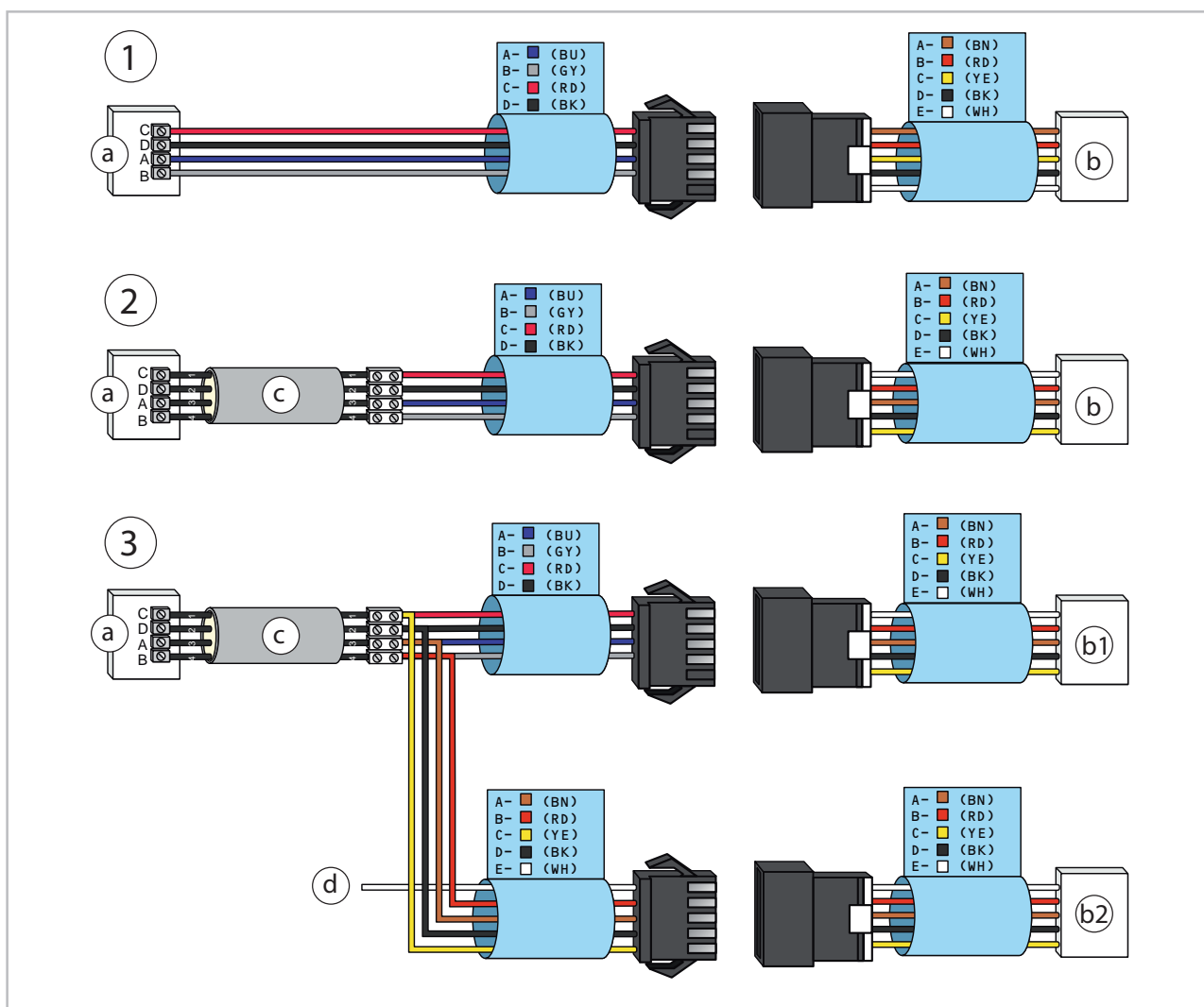
Abb. 4: Elektrisches Anschlussschema
