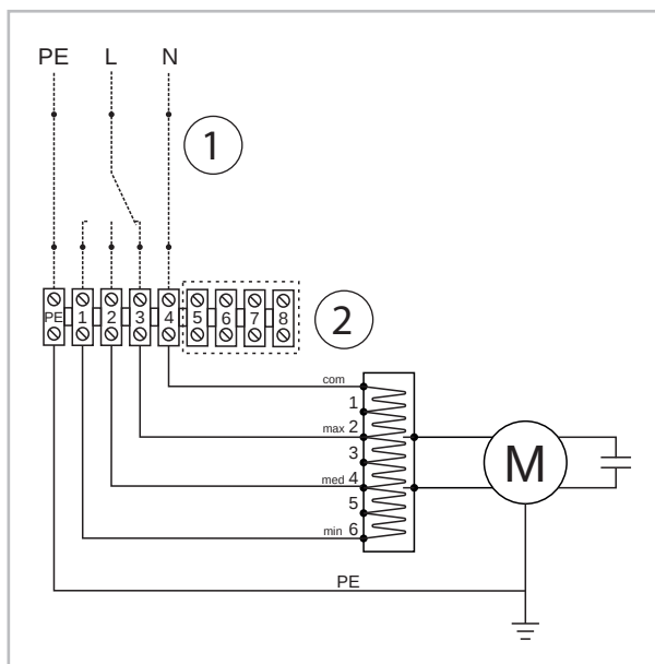
Abb. 17: Elektrisches Schaltschema
