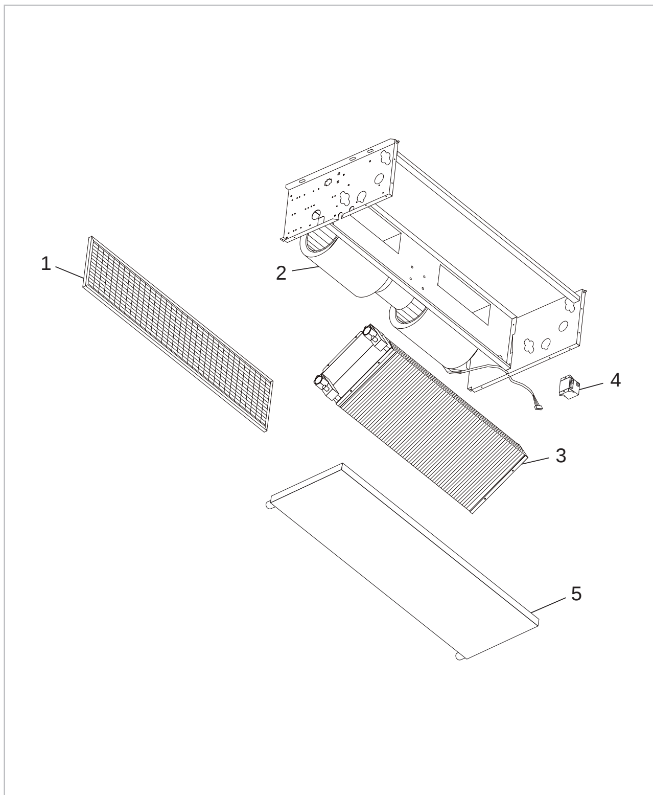
Abb. 22: Gerätedarstellung
