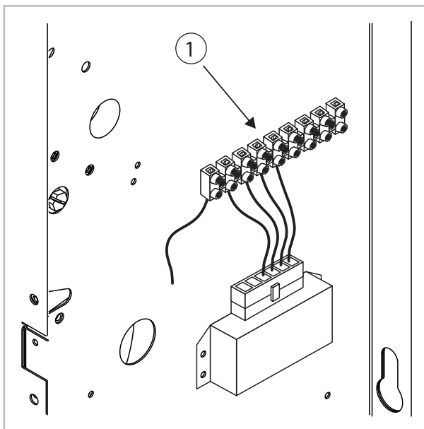
Abb. 16: Elektrischer Anschluss
