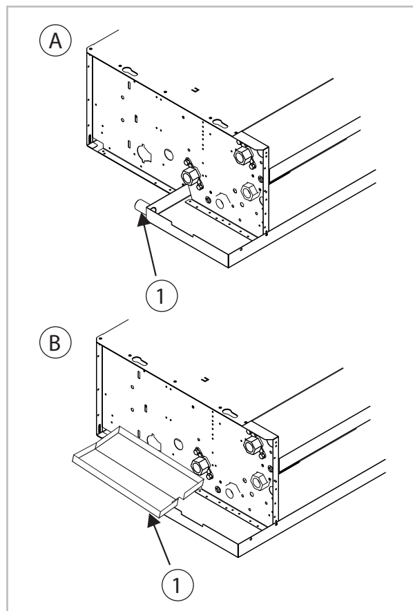
Abb. 15: Kondensatanschluss
