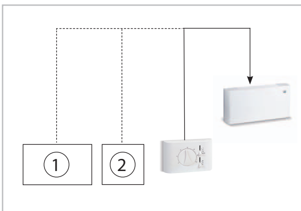
Abb. 10: Einzelansteuerung
