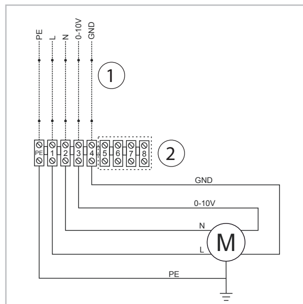
Abb. 17: Elektrisches Schaltschema
