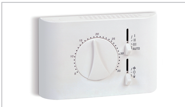
Abb. 9: Raumtemperatur-Regelung - Aufputzmontage
