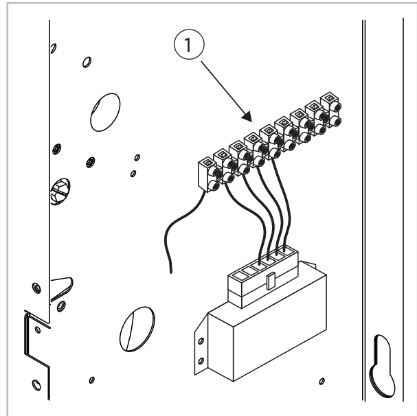
Abb. 16: Elektrischer Anschluss
