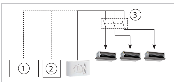
Abb. 11: Gruppenansteuerung
