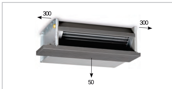
Abb. 11: Mindestfreiräume KWK 135 - KWK 875 ZW (alle Angaben in mm)
