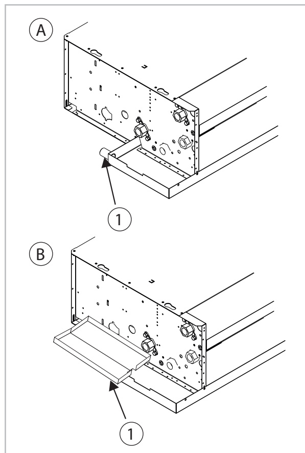
Abb. 15: Kondensatanschluss
