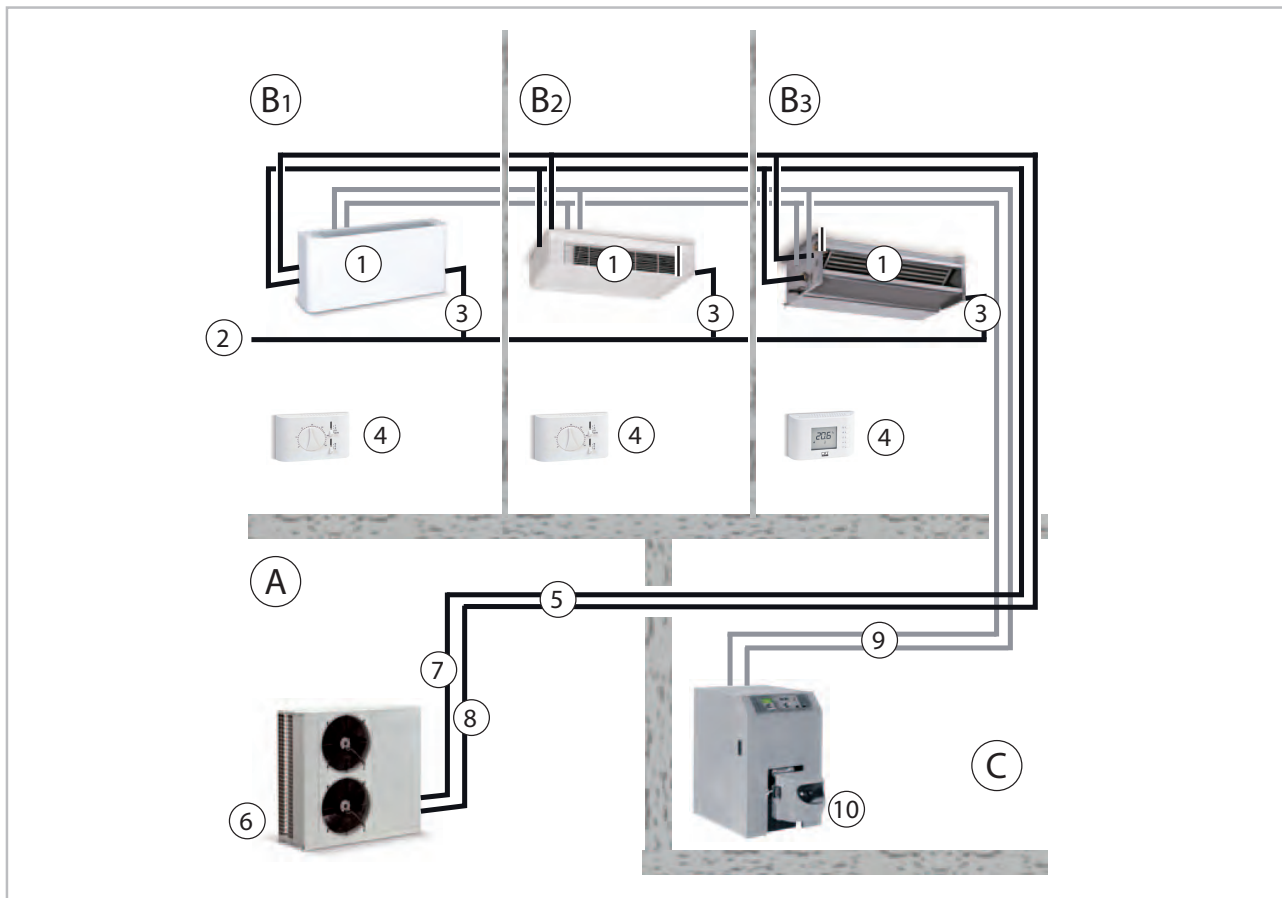
Abb. 5: Beispiel Systemaufbau 4-Leiter-System (Kaltwasser-Klimasystem)
