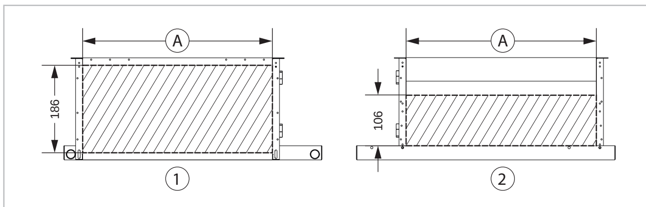
Abb. 13: Abmessungen Kanalanschlüsse
