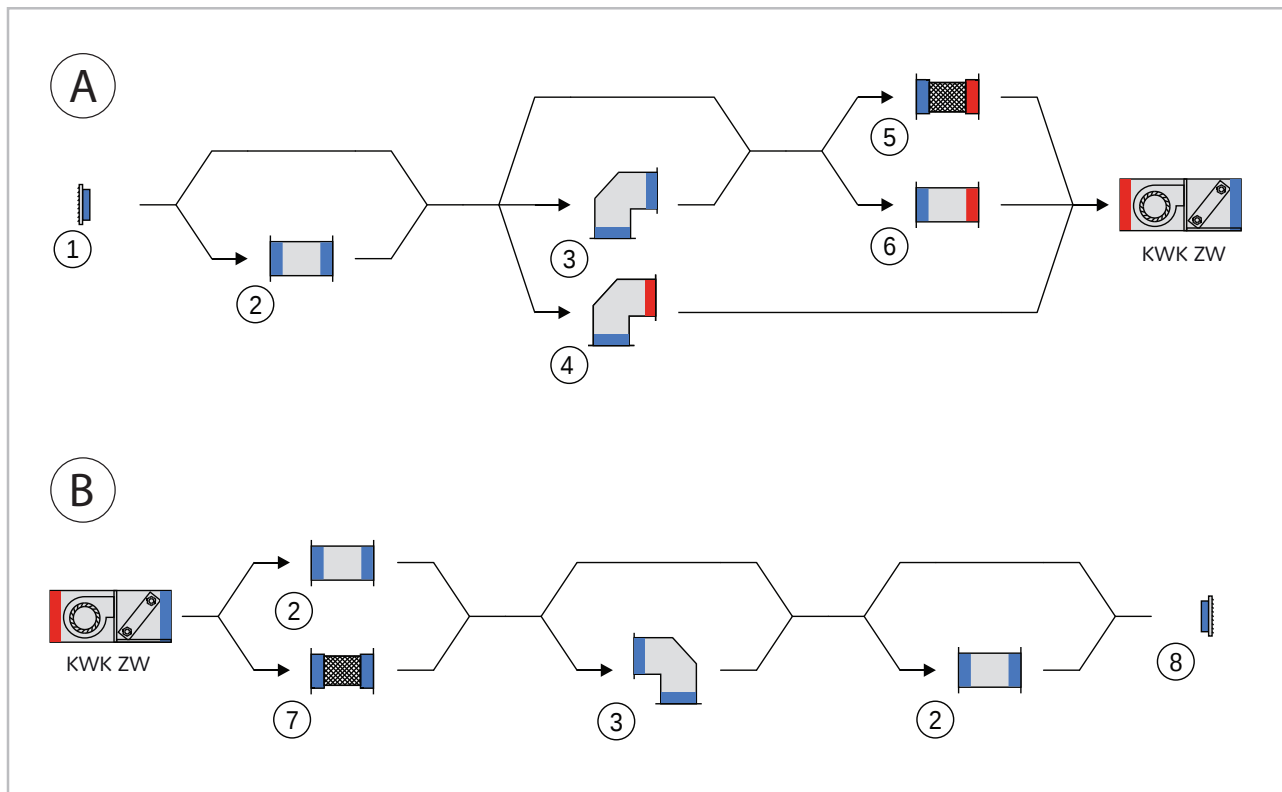
Abb. 12: Luftführung
