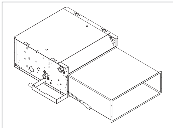
Abb. 14: Montage von Kanalkomponenten
