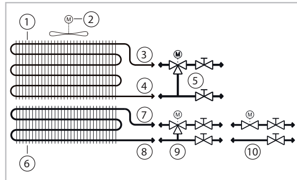
Abb. 3: Schema Mediumkreis 4-Leiter-System (mit Heizregister)
