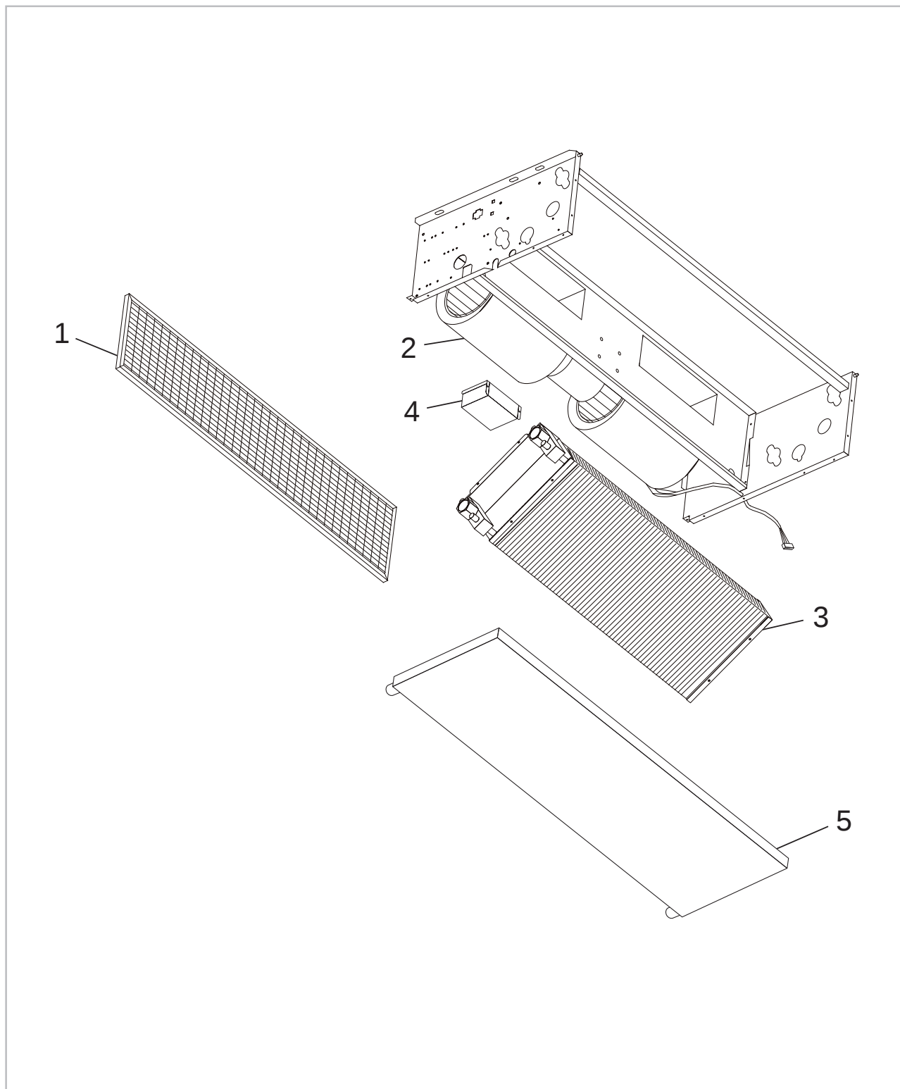
Abb. 22: Gerätedarstellung
