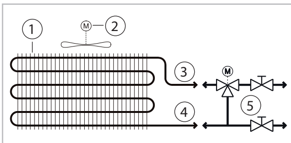
Abb. 2: Schema Mediumkreis 2-Leiter-System
