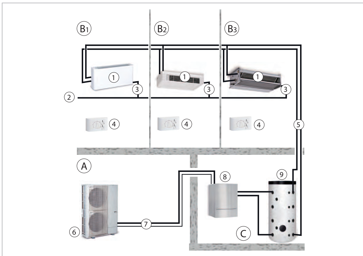
Abb. 4: Beispiel Systemaufbau 2-Leiter-System (Wärmepumpen-System)
