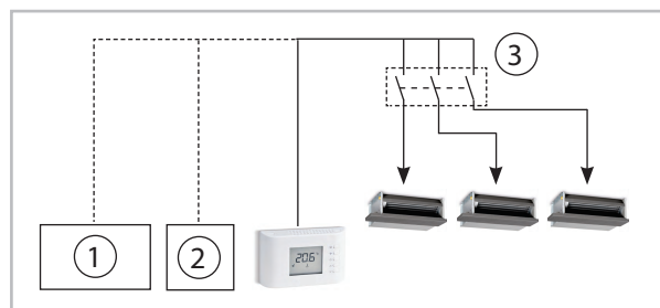
Abb. 9: Gruppenansteuerung
