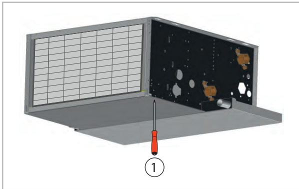
Abb. 21: Demontage Geräteverkleidung
