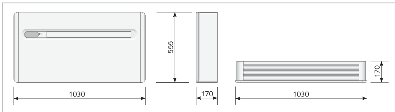
Abb. 1: Geräteabmessungen KWT 240 DC (Alle Angaben in mm)
