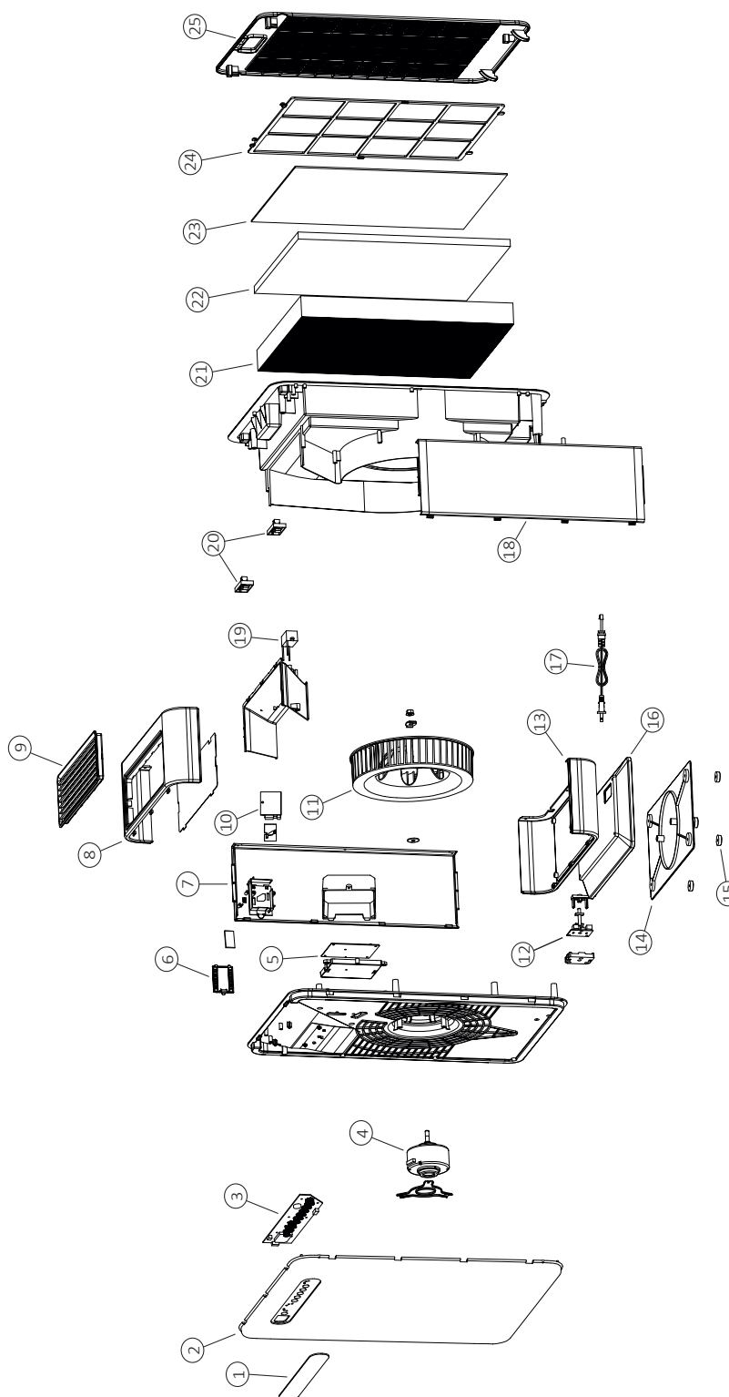
Abb. 18: Explosionszeichnung LRM 350, LRM 500
