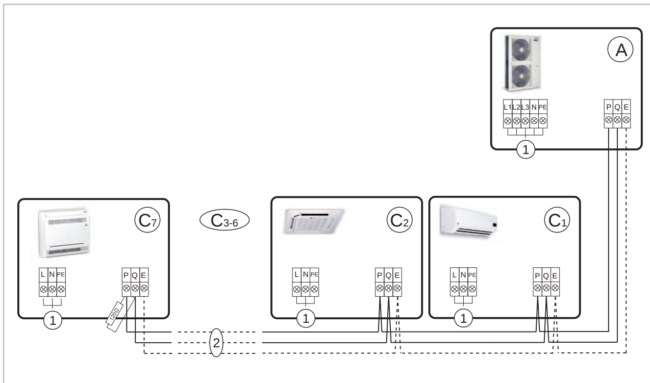
Abb. 19: Elektrisches Anschlussschema
