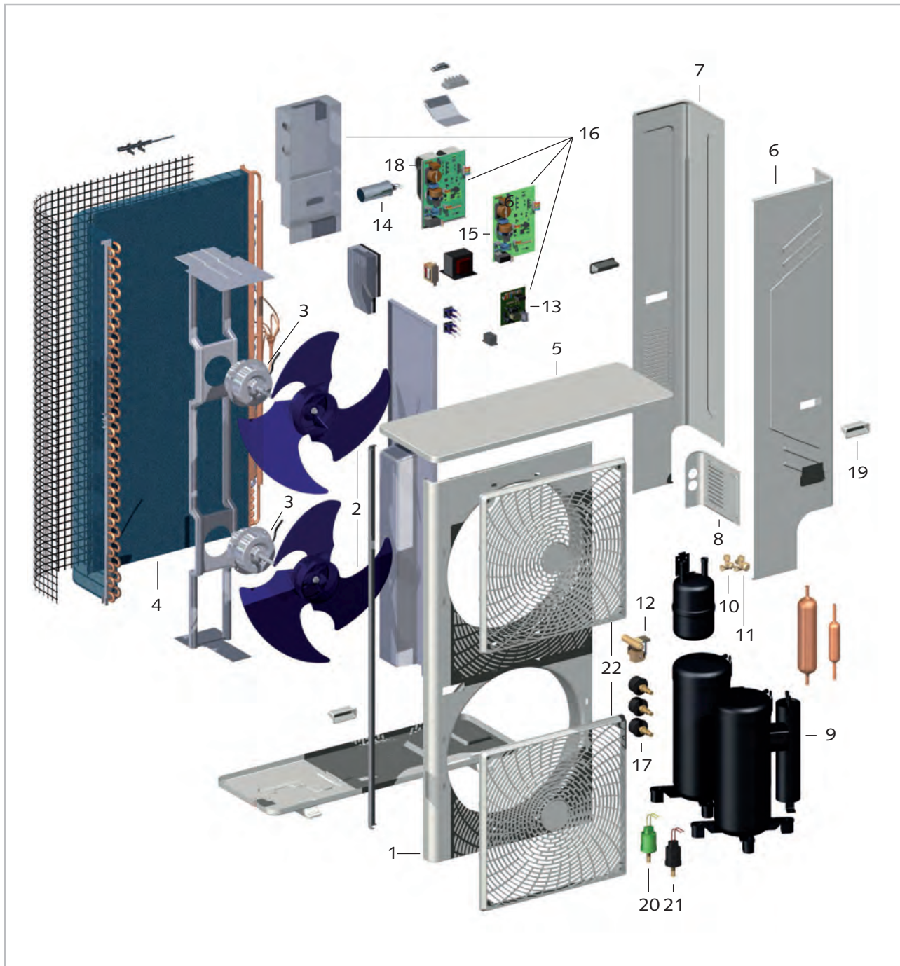
Abb. 39: Gerätedarstellung MVV 1200-2000 DC
