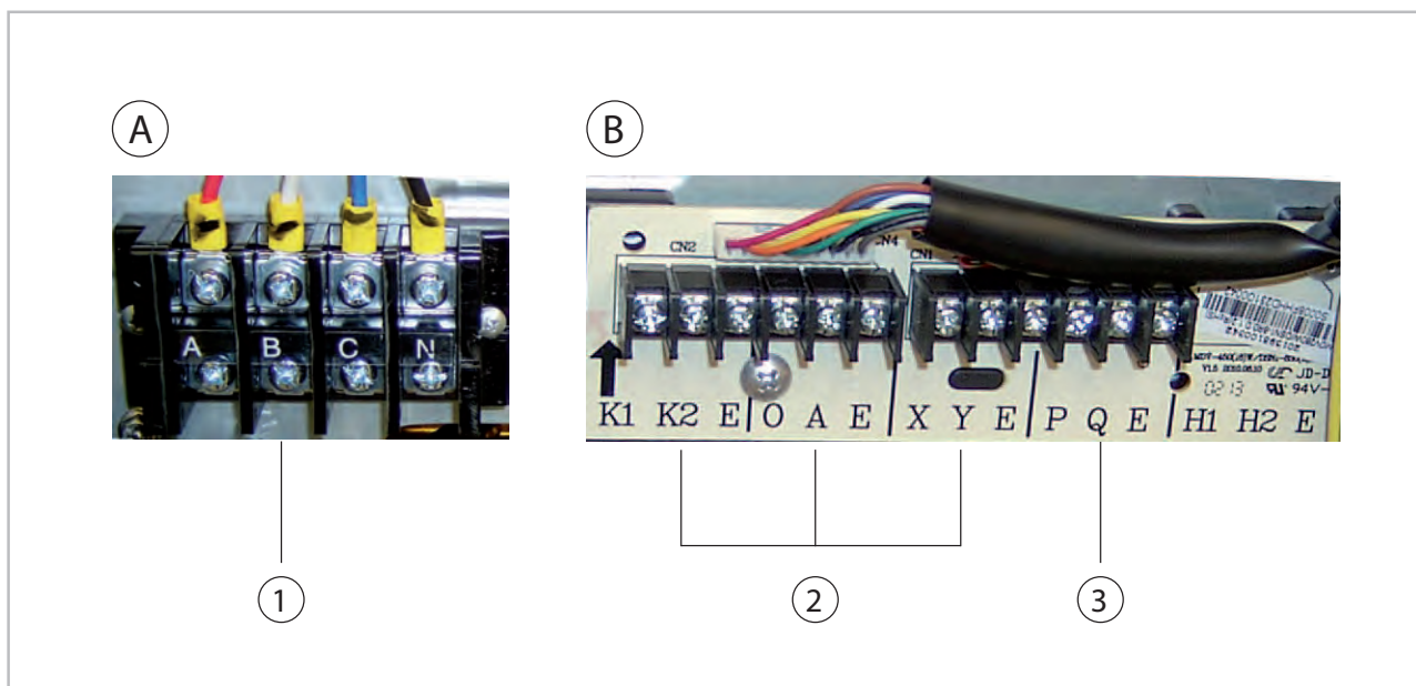
Abb. 29: Elektrischer Anschluss der Leitungen an das Außenteil MVV 2000 DC
