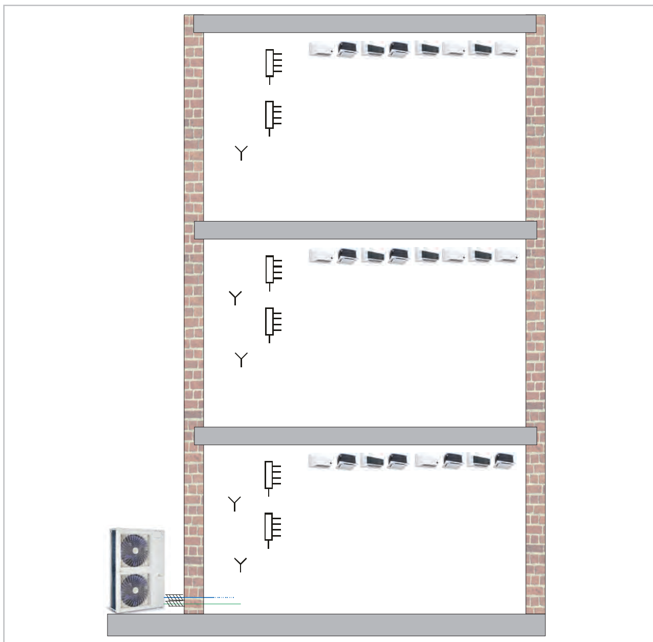
Abb. 23: Skizze zur Ermittlung der nachzufüllenden Kältemittelmenge
