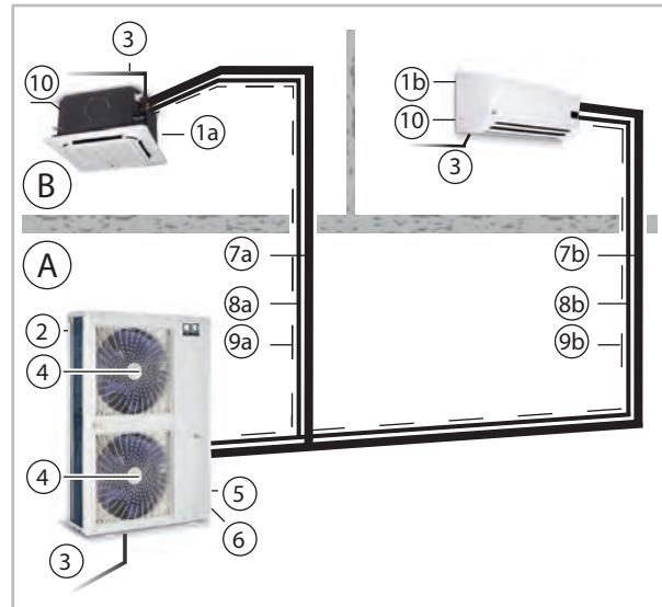
Abb. 7: Systemaufbau
