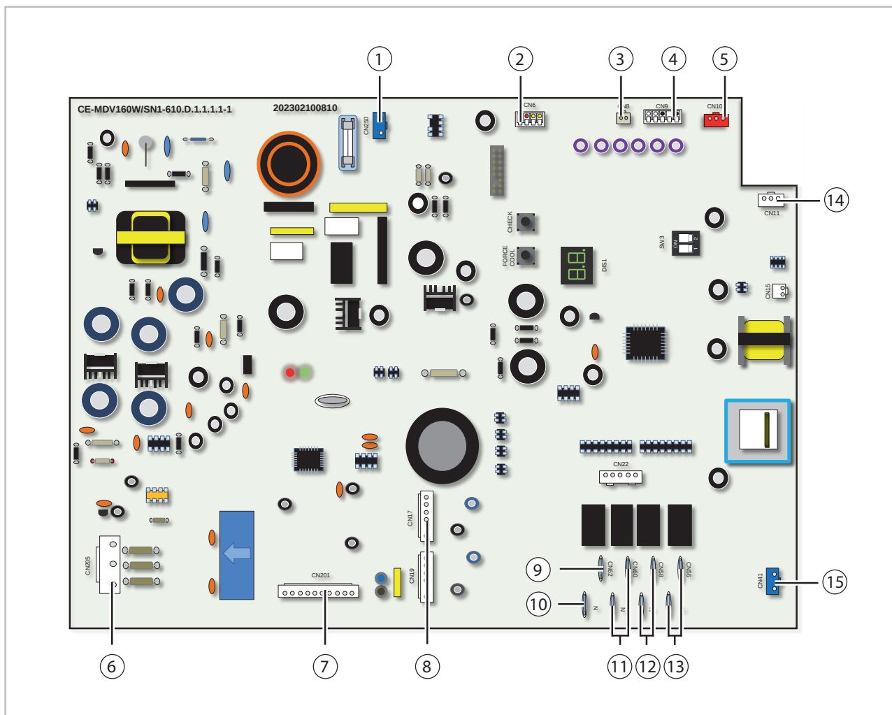
Abb. 31: Elektrisches Schaltschema MVV 1200 DC - Steuerplatine
