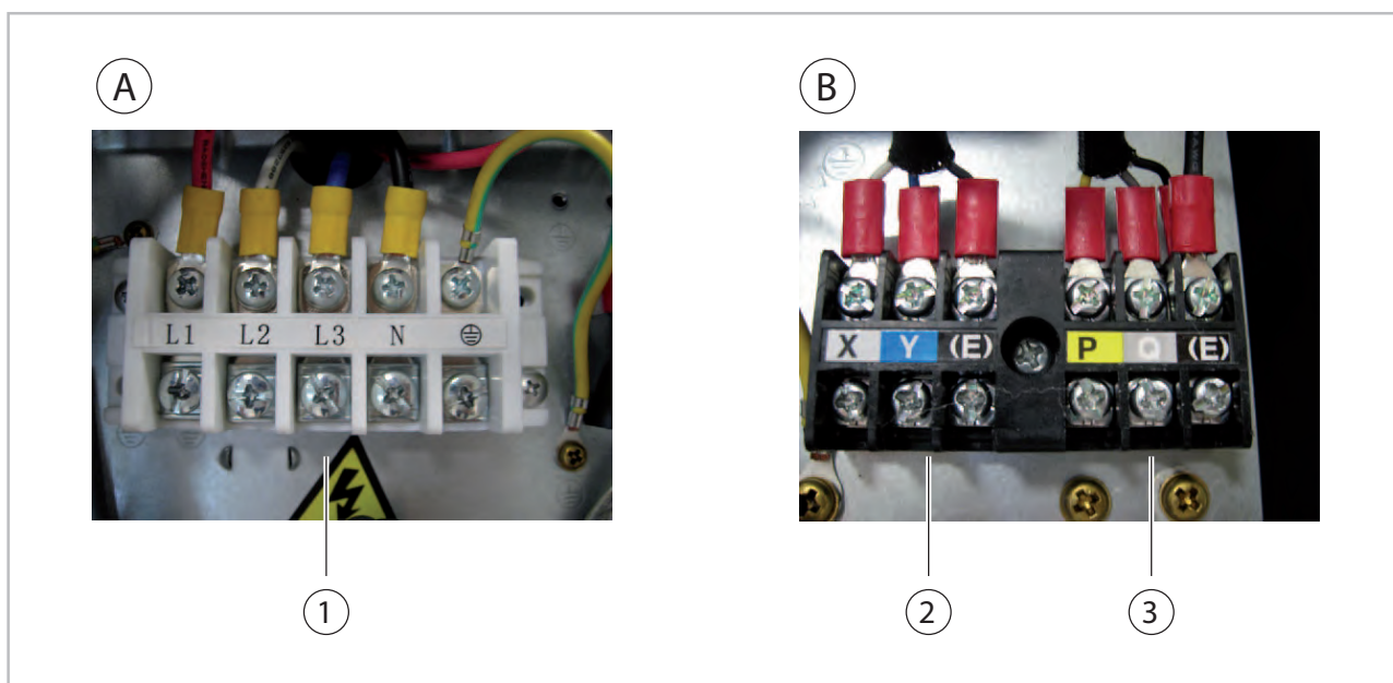
Abb. 28: Elektrischer Anschluss der Leitungen an die Außenteile MVV 1200-1600 DC
