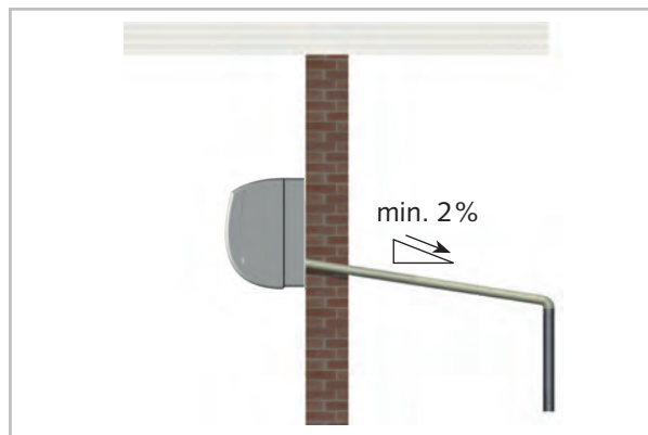
Abb. 17: Kondensatanschluss
