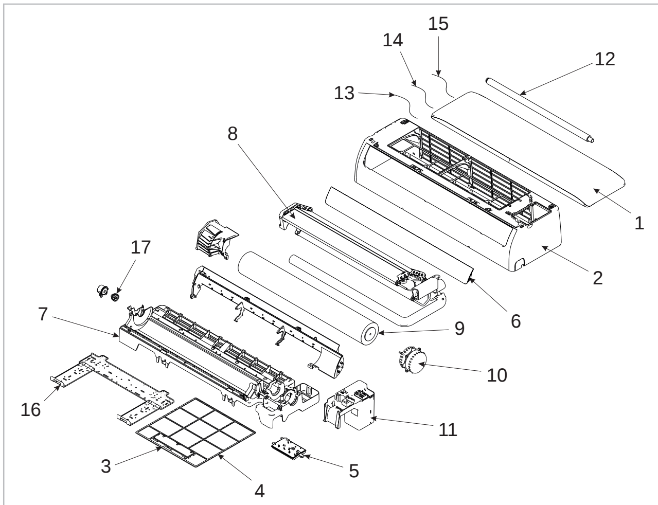
Abb. 25: Gerätedarstellung MVW 222-562
