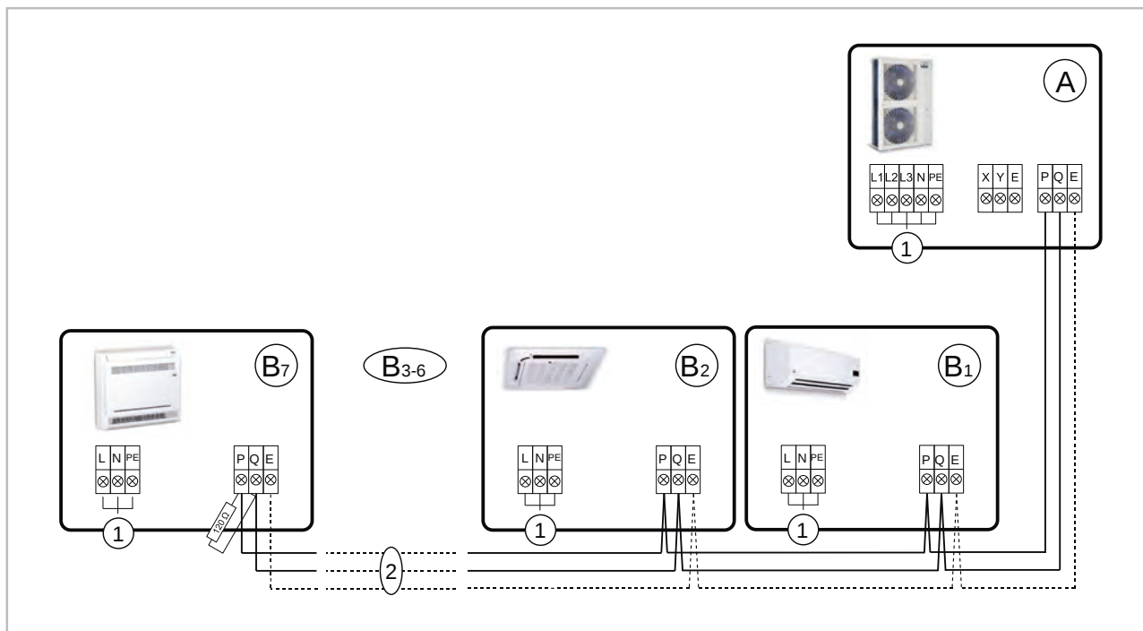
Abb. 19: Elektrisches Anschlussschema
