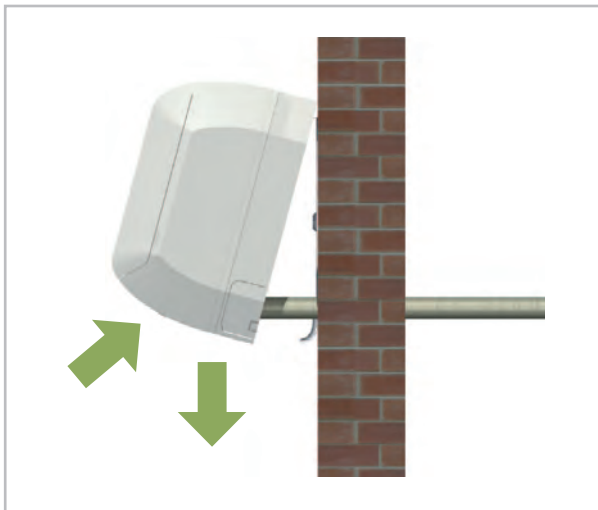
Abb. 14: Waagerechte Ausrichtung
