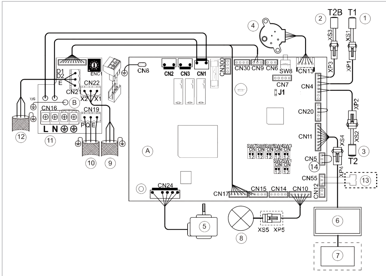
Abb. 20: Elektrisches Schaltschema
