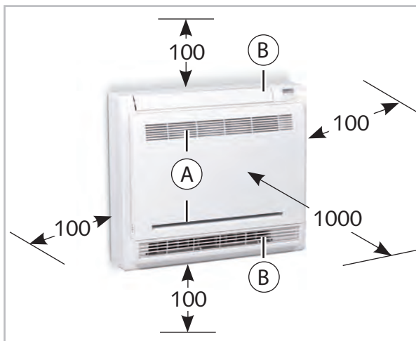
Abb. 11: Mindestfreiräume (alle Angaben in mm)
