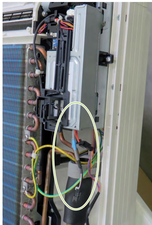
Abb. 4: Anschluss KFB-3
