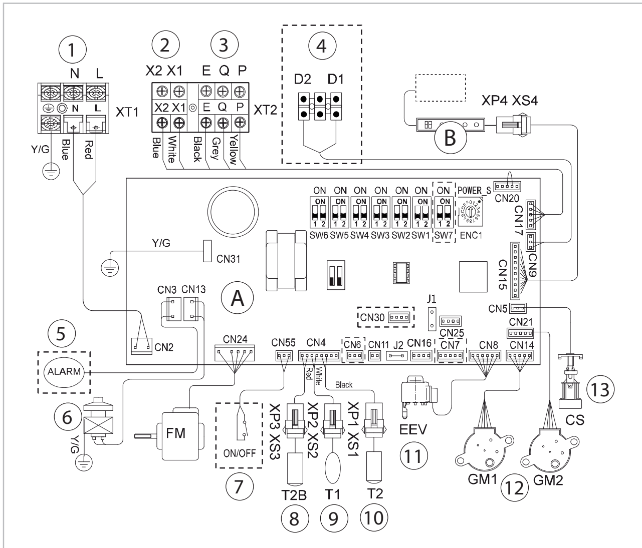
Abb. 18: Elektrisches Schaltschema
