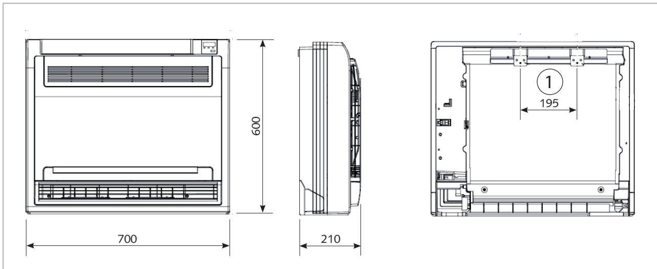
Abb. 1: Geräteabmessungen MXV 221-451 (Alle Angaben in mm)
