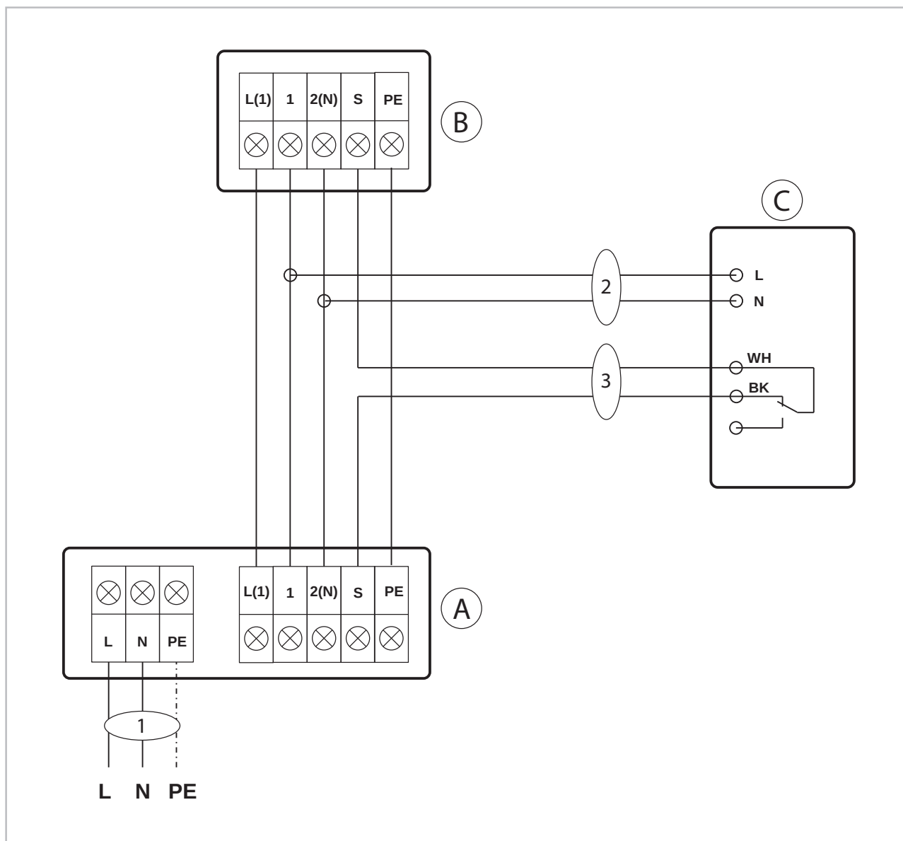
Abb. 17: Elektrisches Anschlussschema
