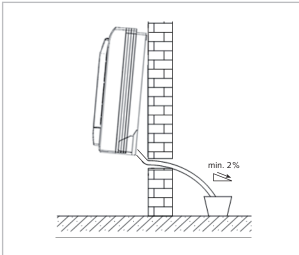
Abb. 14: Kondensatanschluss
