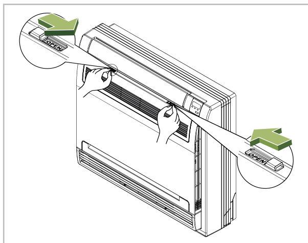
Abb. 7: Vorderwand öffnen
