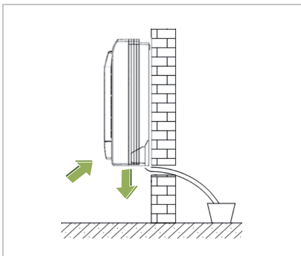
Abb. 13: Waagerechte Ausrichtung
