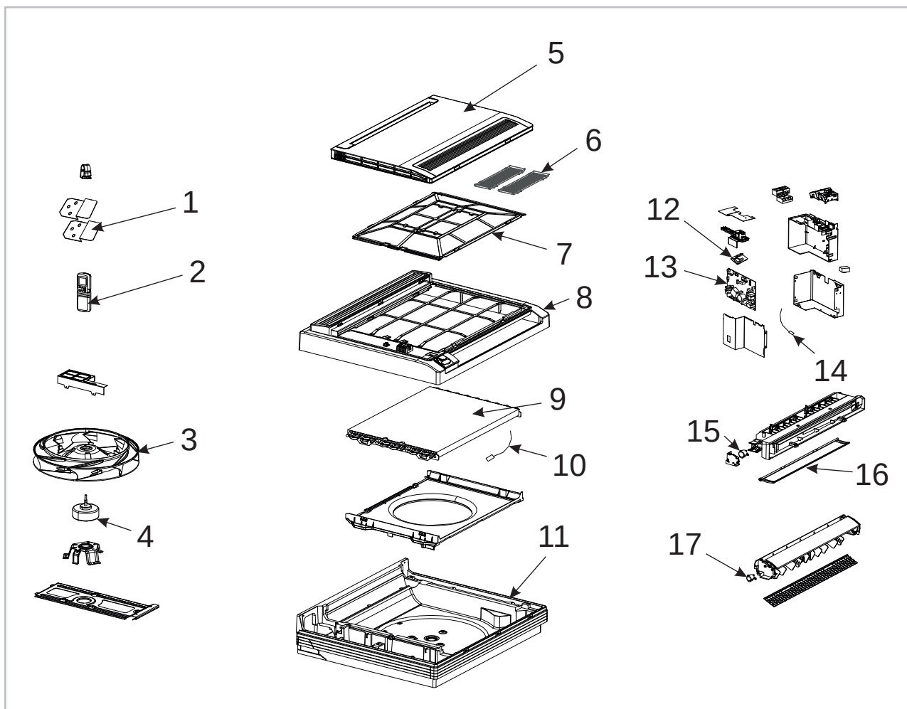
Abb. 22: Explosionszeichnung
