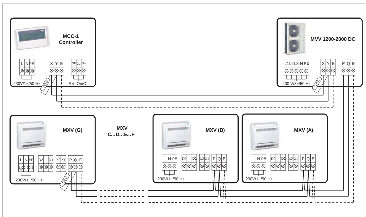
Abb. 16: Elektrisches Anschlussschema
