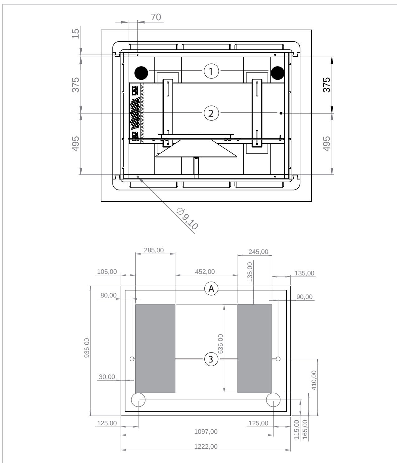
Abb. 10: Streifenfundament SWK 5.1 und SWK 7.1
