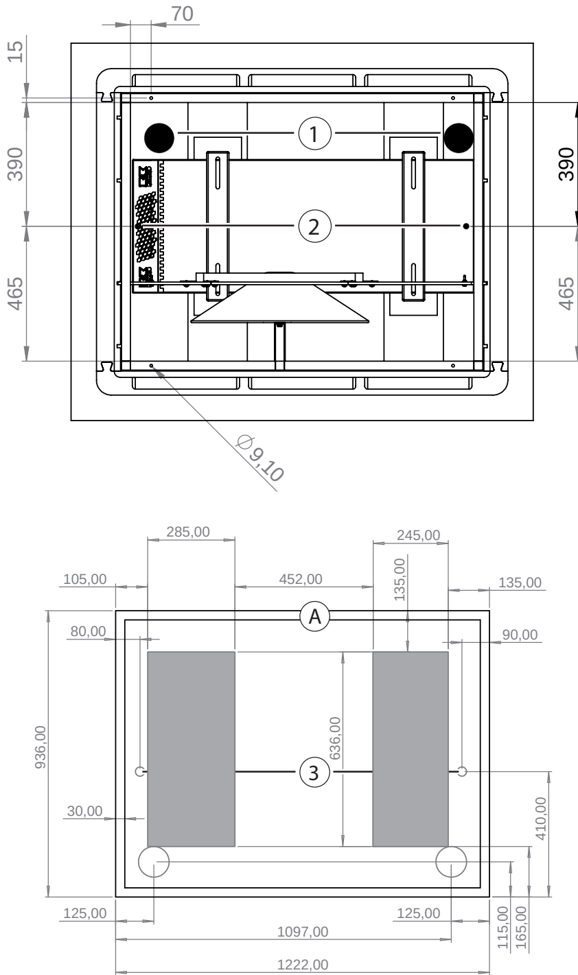
Abb. 9: Streifenfundament SWK 4.1
