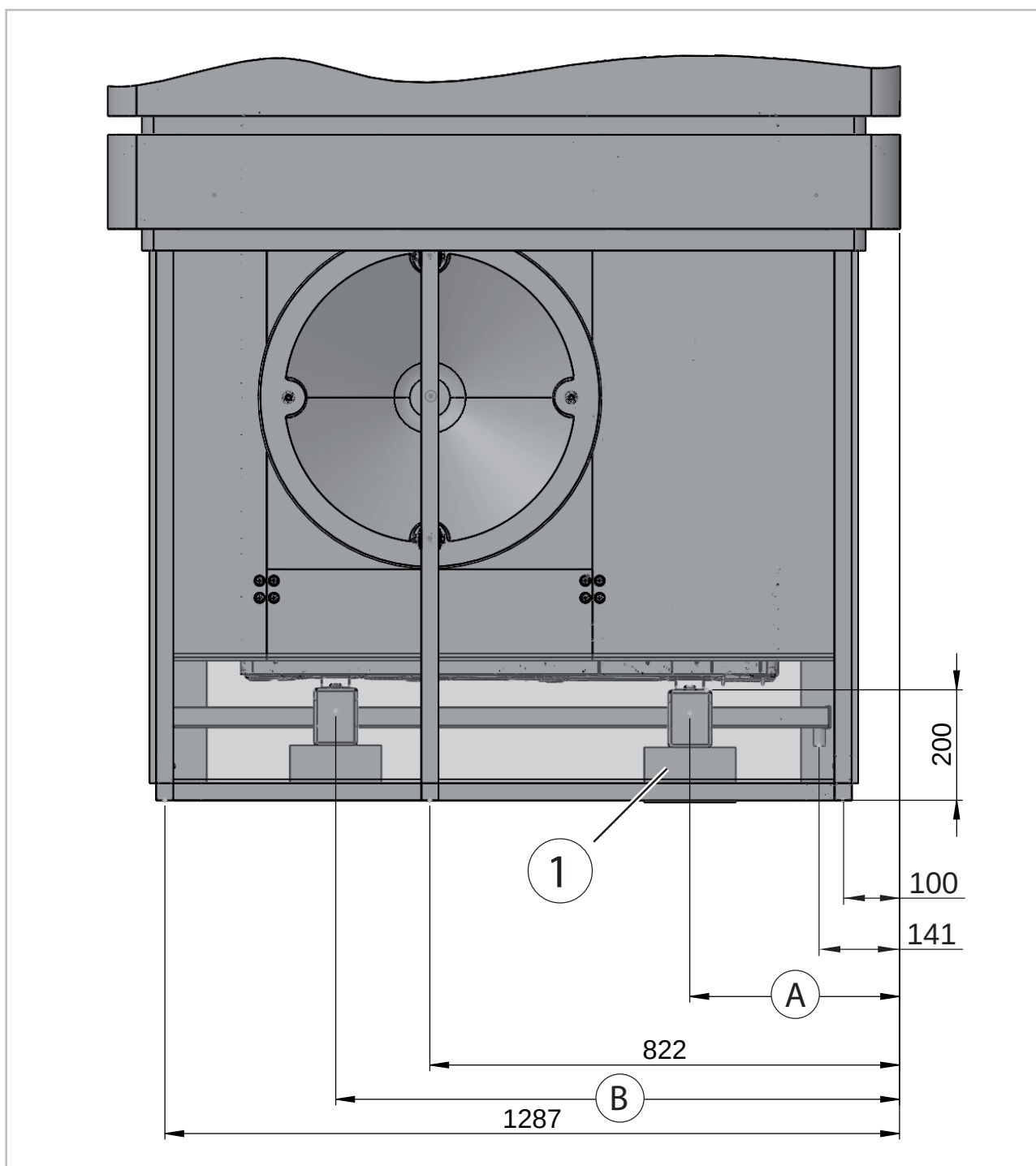
Abb. 3: Vorderansicht Schallschutzhaube SWK 5.1 und SWK 7.1 (Alle Maße in mm)
