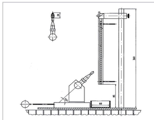
Abb. 5: Aufbau zur vertikalen Beflammung der Probekörper
