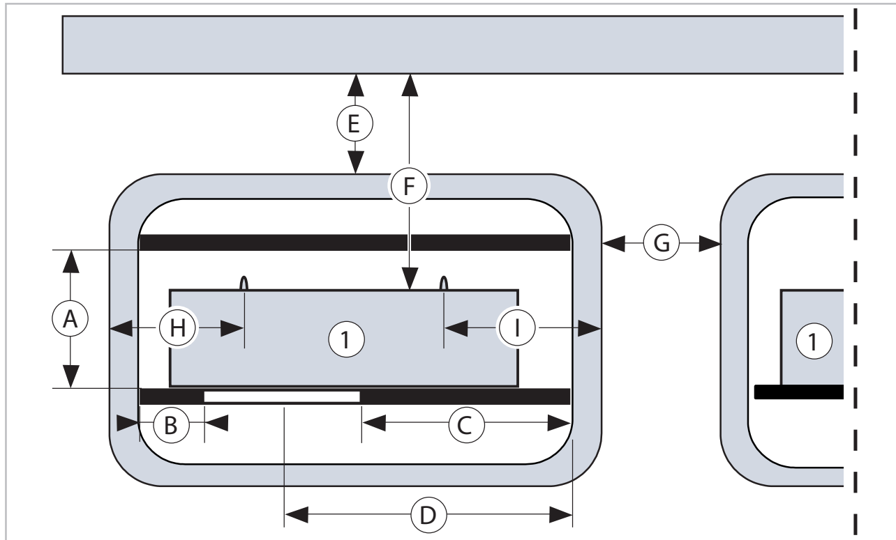
Abb. 4: Abmessungen Schallschutzhauben mit Außenmodulen (alle Maße in mm)
