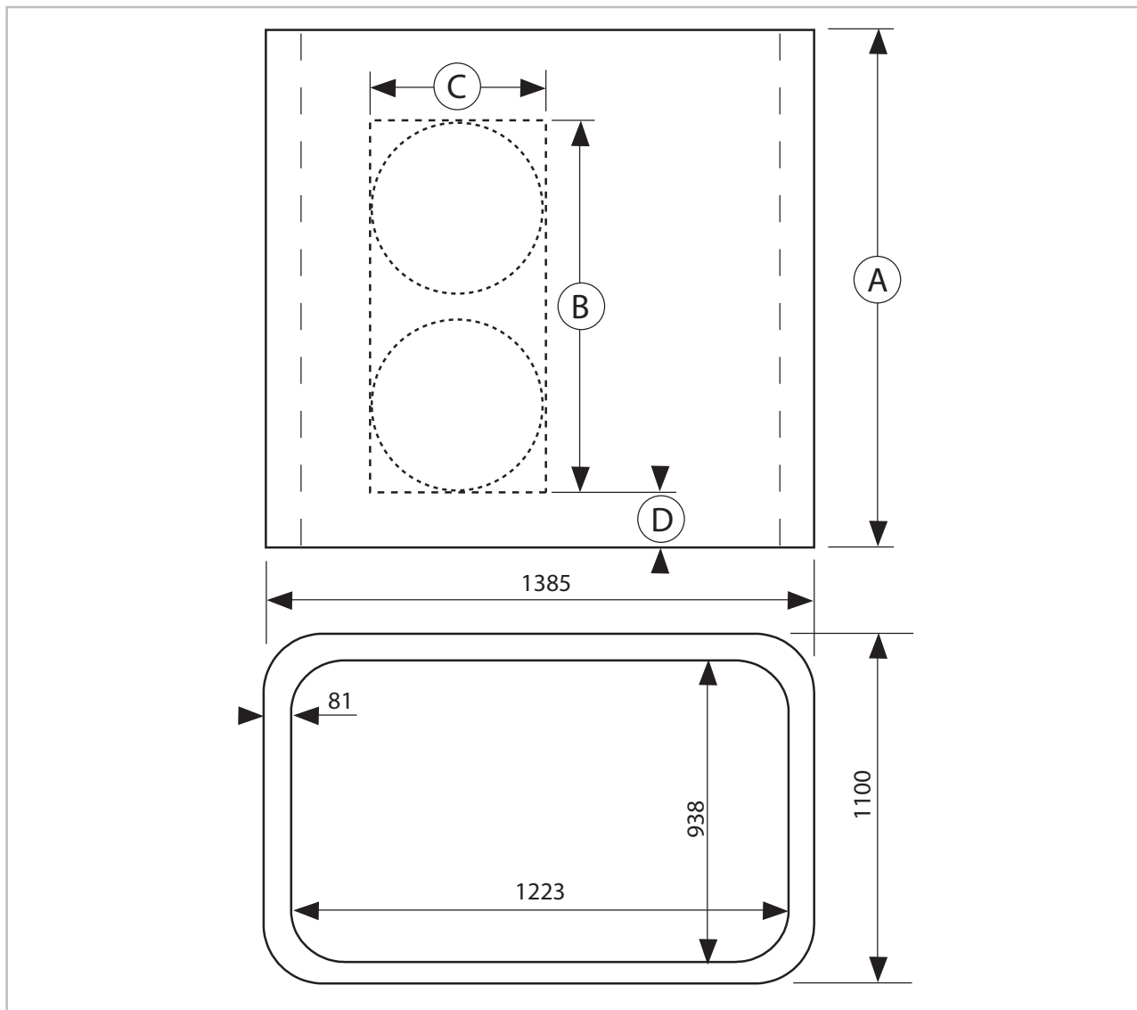
Abb. 1: Abmessungen Schallschutzhauben (Alle Maße in mm)
