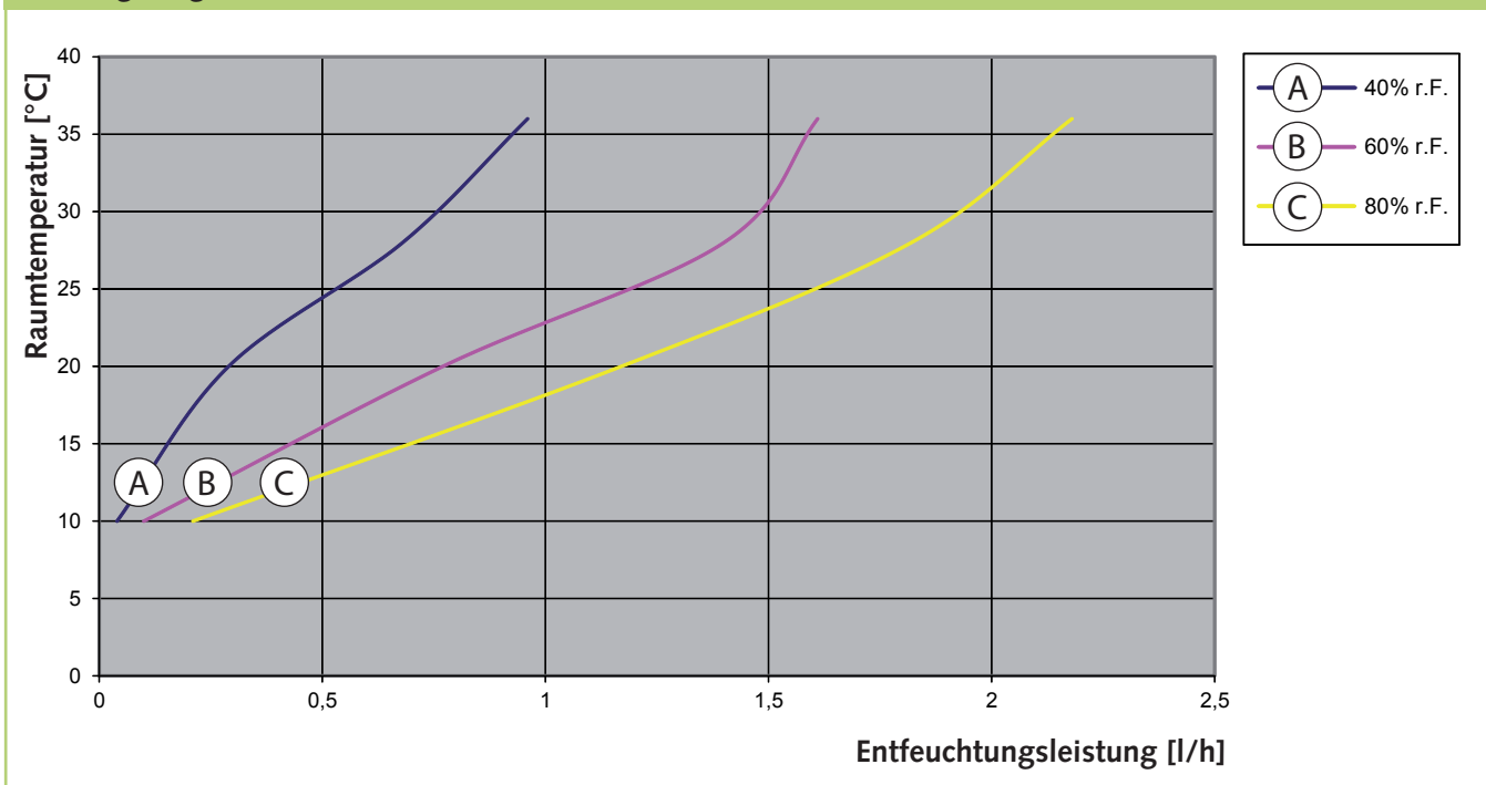
Leistungsdiagramm SLN 45
