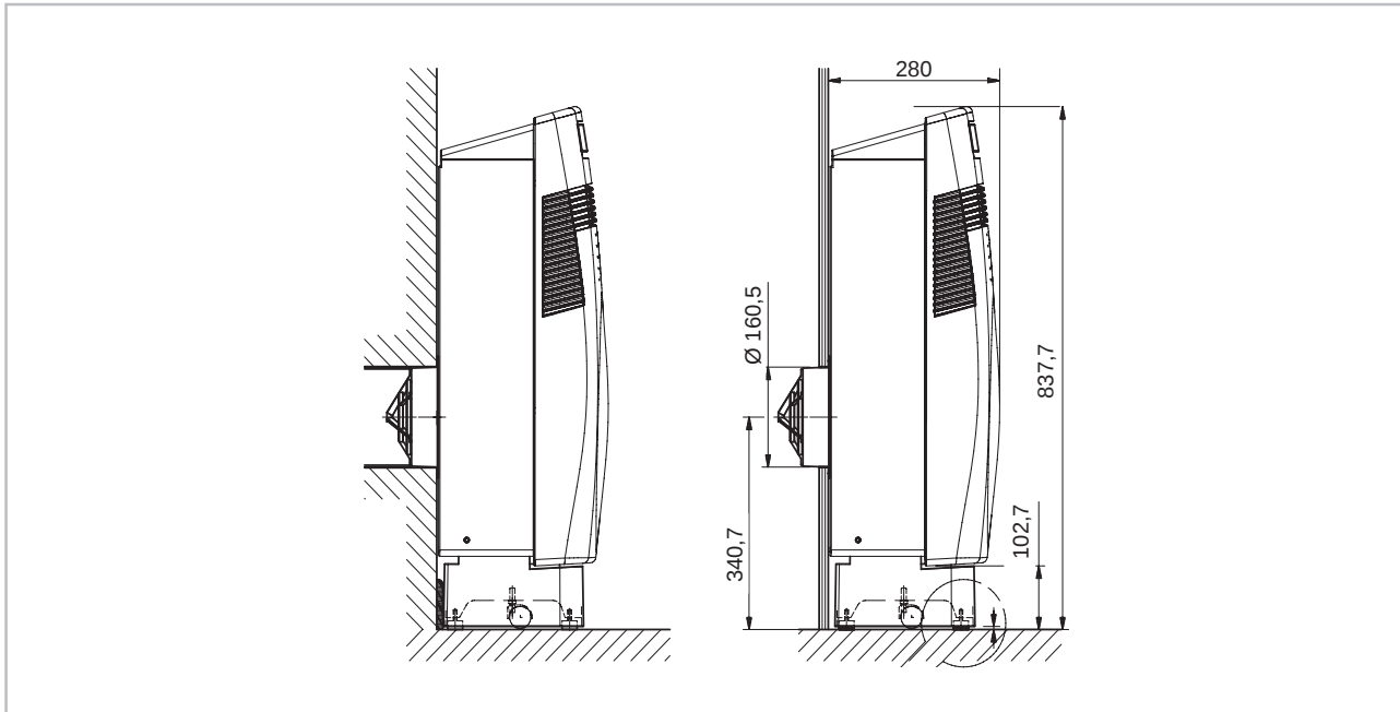
Abb. 1: Abmessungen
