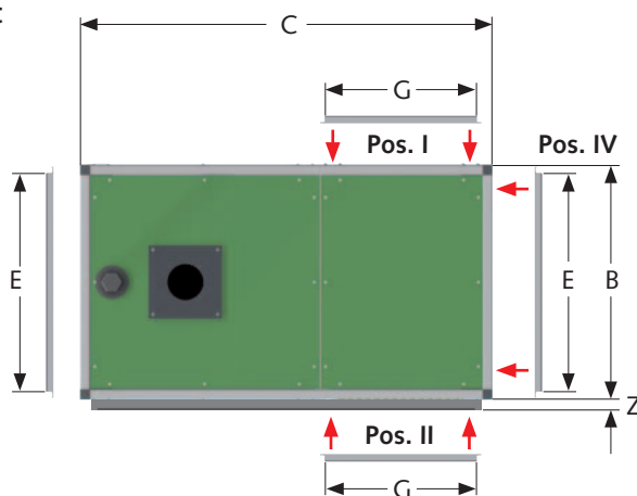
Liegendes Gerät
