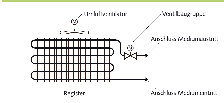
Schema Mediumkreis
