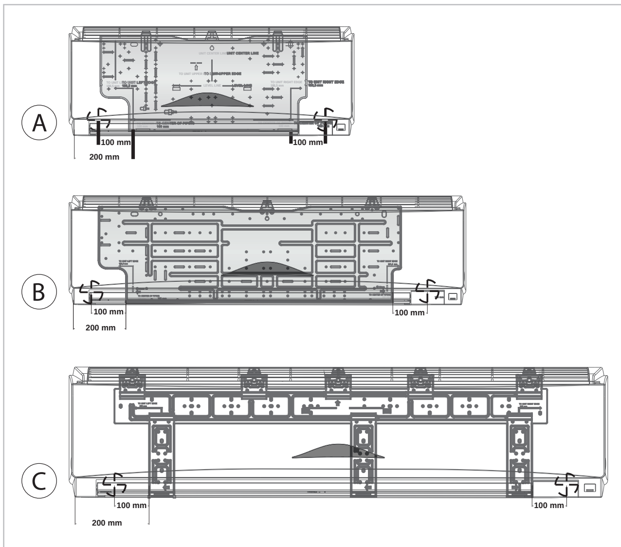
Abb. 10: Montageplatten
