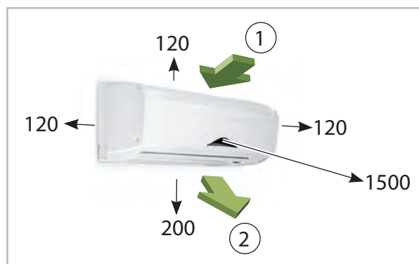
Abb. 8: Mindestfreiräume (alle Angaben in mm)
