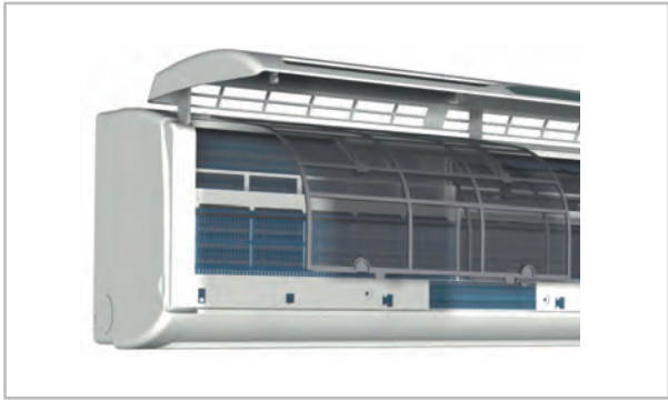
Abb. 18: Gitter nach oben klappen
