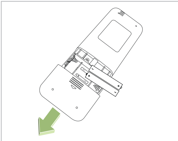
Abb. 6: Einsetzen der Batterien
