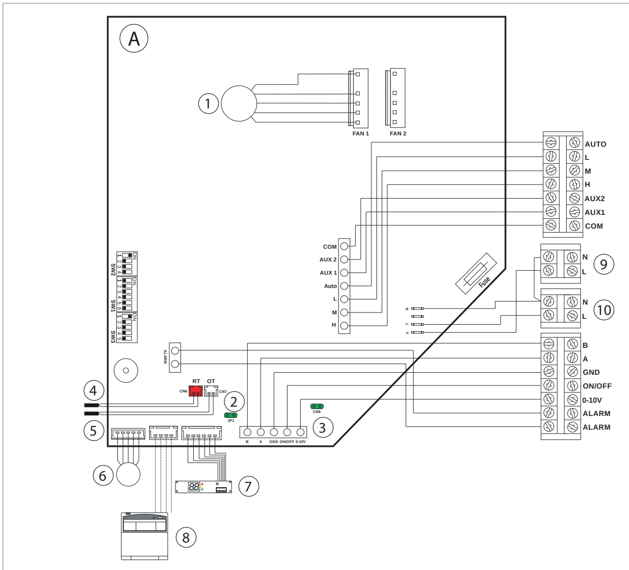
Abb. 15: Elektrisches Schaltschema
