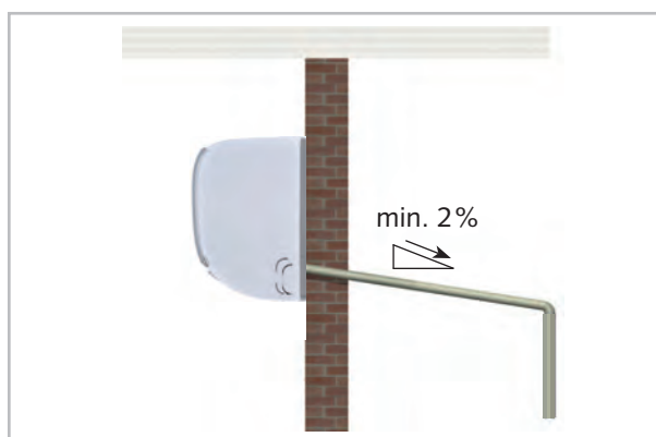
Abb. 12: Kondensatanschluss
