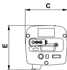
ÖWAMAT 12 - 14 ohne Vorabscheidevorrichtung without preseparation sans citerne de précollecte zonder vóór-afscheidingsinstallatie
