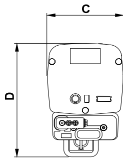
ÖWAMAT 12 - 14 mit Vorabscheidevorrichtung with preseparation avec citerne de précollecte met vóór-afscheidingsinstallatie
