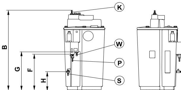
ÖWAMAT 12 - 14 ohne Vorabscheidevorrichtung without preseparation sans citerne de précollecte zonder vóór-afscheidingsinstallatie
