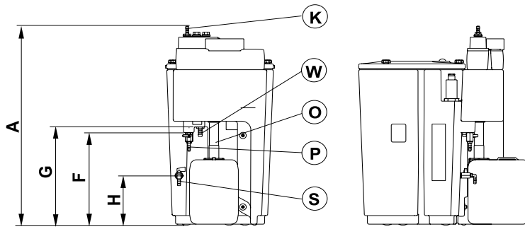
ÖWAMAT 12 - 14 mit Vorabscheidevorrichtung with preseparation avec citerne de précollecte met vóór-afscheidingsinstallatie
